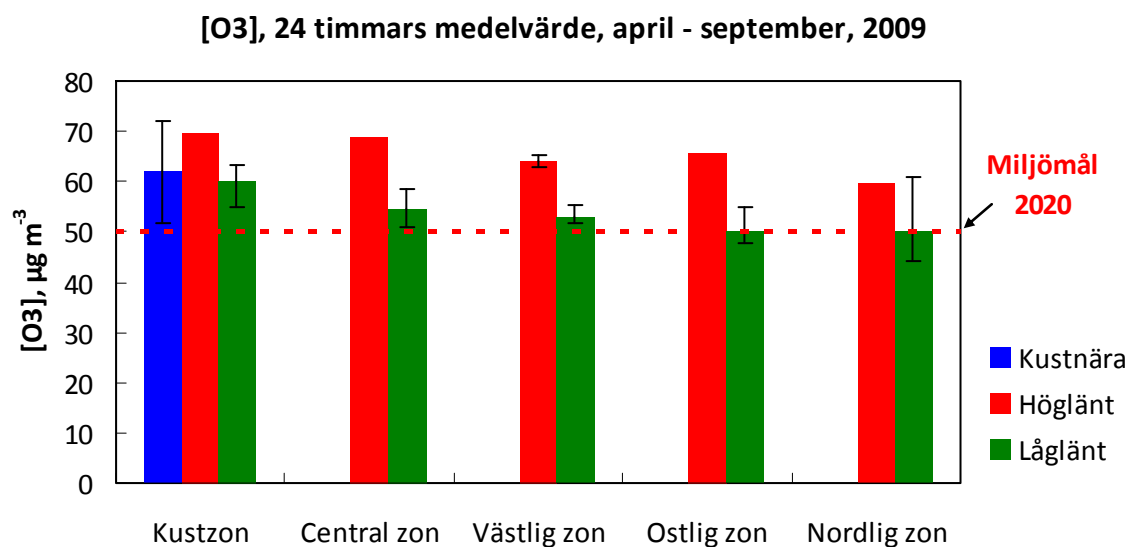
Figur 17. Genomsnittliga ozonkoncentrationer som 24-timmars medelvärde för perioden april-september 2009 och fördelade på de zoner som ingår i mätprogrammet. De tunna svarta staplarna indikerar det maximala och minimala värdet inom respektive kategori, när antalet mätplatser är flera än två.
