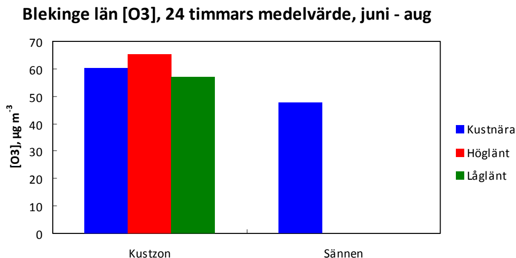
Figur 25. Genomsnittliga ozonkoncentrationer för i Blekinge relevant zon samt för samtliga stationer i länet under juni – augusti 2009.
