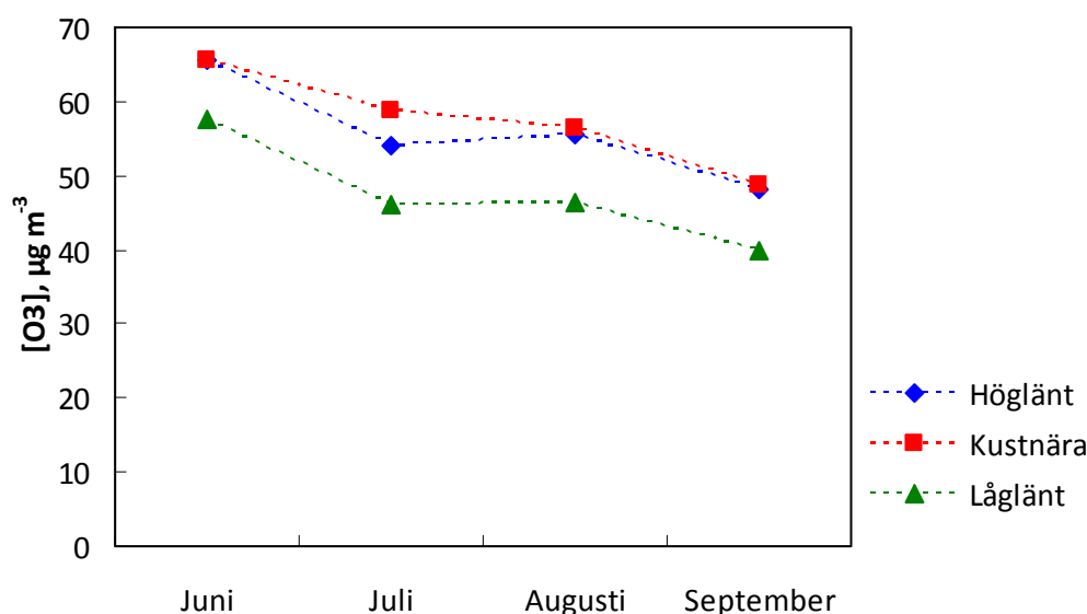
Figur 12. Genomsnittliga månadsvisa ozonhalter (juni – september) observerade under 2009 inom Ozonmättnätet uppdelade på lokaltyperna kustnära, höglänt och låglänt. Klintaskogen, Draftinge, Hoburgen, Ålleberg och Lanna saknar O_3 -data för september månad.
