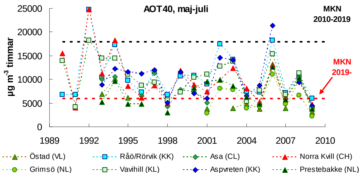
Figur 8. Årsvisa värden för 12 timmars AOT40 1 maj – 31 jul vid platser i södra Sverige med timvisa instrumentmätningar av ozonhalter inom den nationella miljöövervakningen, en norsk EMEP-station, samt i regi av IVL (Östad) och SLU (Asa). Gröna punkter indikerar låglänta, röda höglänta och blå kustnära mätlokaler.
