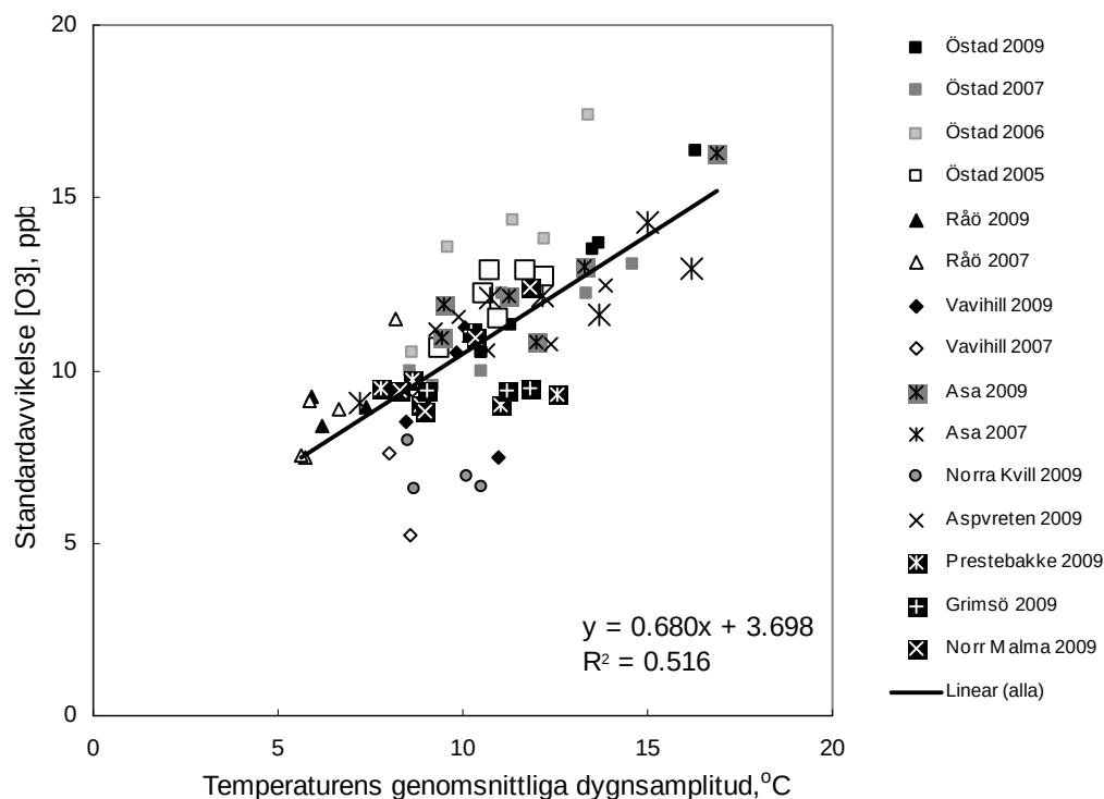
Figur 3. Samband mellan standardavvikelse för timvisa ozonhalter och temperaturens genomsnittliga dygnsamplitud för stationer med kontinuerligt registrerande instrument för ozon. Figuren innehåller data för 2009 och för tidigare år för några mätplatser.
