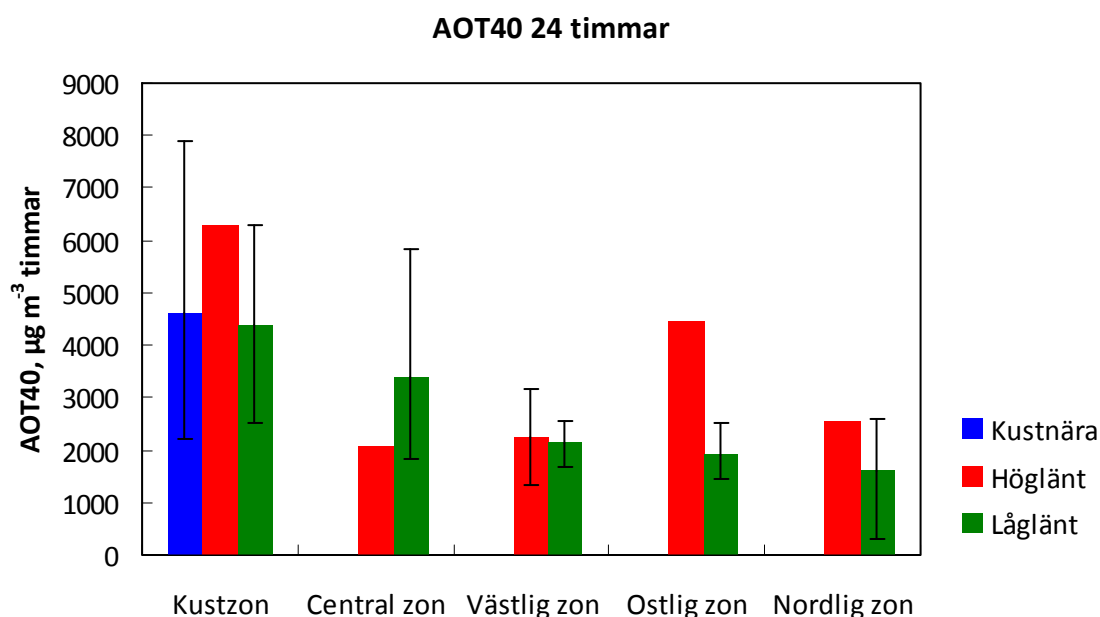
Figur 15. Ozonindex inom Ozonmättnätet för 24 timmars AOT40 för perioden juni-augusti 2009 och fördelade på zon inom mätprogrammet. De tunna svarta staplarna indikerar det maximala och minimala värdet inom respektive kategori, när antalet mätplatser är flera än två.
