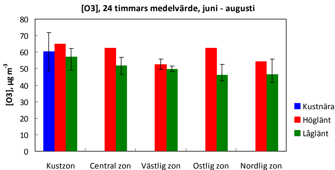
Figur 13. Genomsnittliga ozonkoncentrationer för samtliga stationer inom ozonmättnätet under juni – augusti 2009 fördelade på de zoner och kategorier som ingår i mätprogrammet. De tunna svarta staplarna indikerar det maximala och minimala värdet inom respektive kategori, när antalet mätplatser är fler än en.
