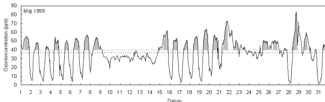
Figur 1. Ozonhalten mätt på 1 m höjd vid Östad säteri, som ligger i ett låglänt jordbrukslandskap i Västra Götalands län. Den streckade linjen visar medelvärde för perioden. Den grå linjen visar tröskelvärdet 40 ppb och den skuggade arean representerar överskridandet av 40 ppb under dagtid (AOT40). För perioden i figuren var AOT40 = 2\,409 ppb-timmar ( 4818 \mu\text{g}/\text{m}^3 timmar).
