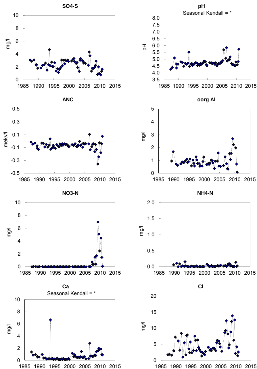
Figur 48. Markvattenkemi vid Knapanäs, G 09 : sulfatsvavel ( \text{SO}_4\text{-S} ), pH, markvattnets syranneutraliserande förmåga (ANC), oorganiskt aluminium (oorg Al), nitratkväve ( \text{NO}_3\text{-N} ), ammoniumkväve ( \text{NH}_4\text{-N} ), kalciumhalt ( \text{Ca}^{2+} ) samt klorid (Cl). Saknade värden innebär oftast att marken varit för torr. Trendanalys har genomförts med hjälp av Seasonal-Kendall och signifikansnivåer anges, ovanför respektive diagram, i de fall där signifikanta trender påvisats.
