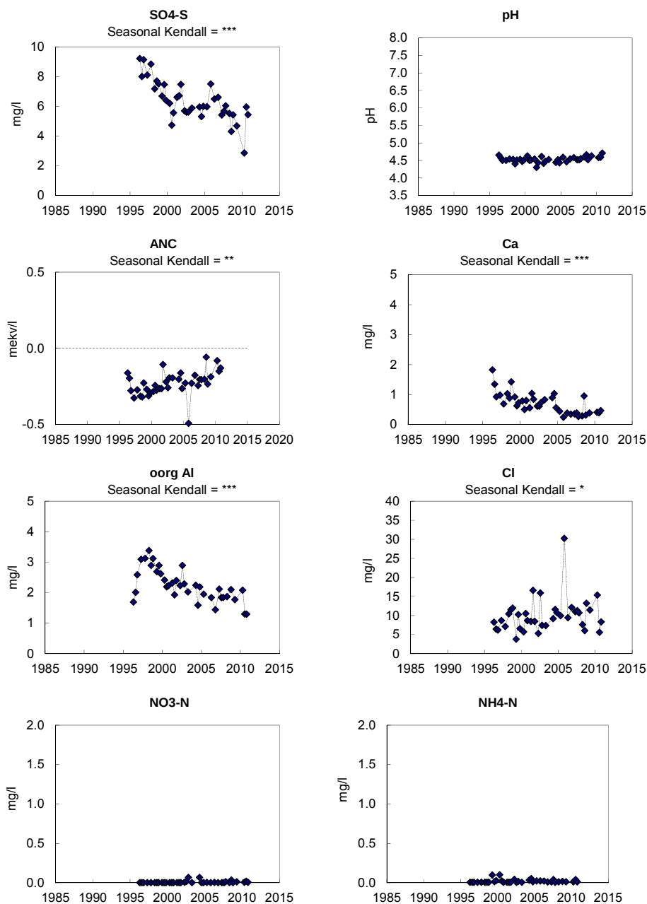
Figur 45. Markvattenkemi vid Vång, K 13. Sulfatsvavel ( \text{SO}_4\text{-S} ); pH; markvattnets syraneutraliserande förmåga (ANC); kalciumhalt (Ca); oorganiskt aluminium (oorg Al); klorid (Cl); nitratkväve ( \text{NO}_3\text{-N} ) samt ammoniumkväve ( \text{NH}_4\text{-N} ). Saknade värden innebär oftast att marken varit för torr. Trendanalys har genomförts med hjälp av Seasonal-Kendall metodik och signifikansnivåer anges, ovanför respektive diagram, i de fall där signifikanta trender påvisats.
