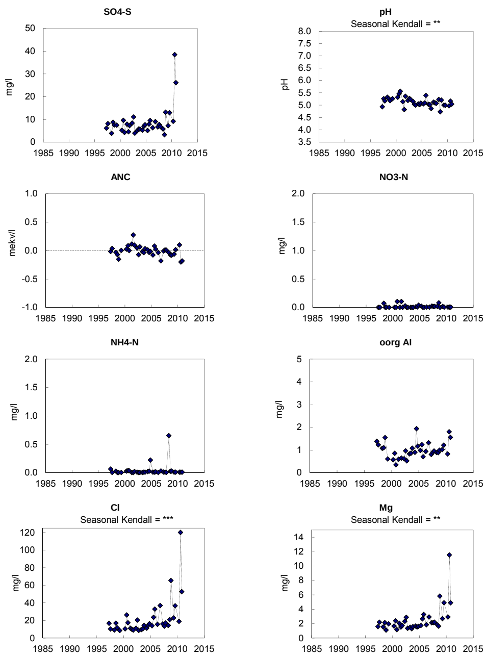
Figur 31. Markvattenkemi vid Rockneby, H 03. Sulfatsvavel ( \text{SO}_4\text{-S} ); pH; markvattnets syraneutraliserande förmåga (ANC); nitratkväve ( \text{NO}_3\text{-N} ); ammoniumkväve ( \text{NH}_4\text{-N} ); oorganiskt aluminium (oorg Al); klorid (Cl) samt magnesium ( \text{Mg}^{2+} ). Saknade värden innebär oftast att marken varit för torr. Trendanalys har genomförts med hjälp av Seasonal Kendall metodik och signifikansnivåer anges ovanför respektive diagram, i de fall där signifikanta trender påvisats.
