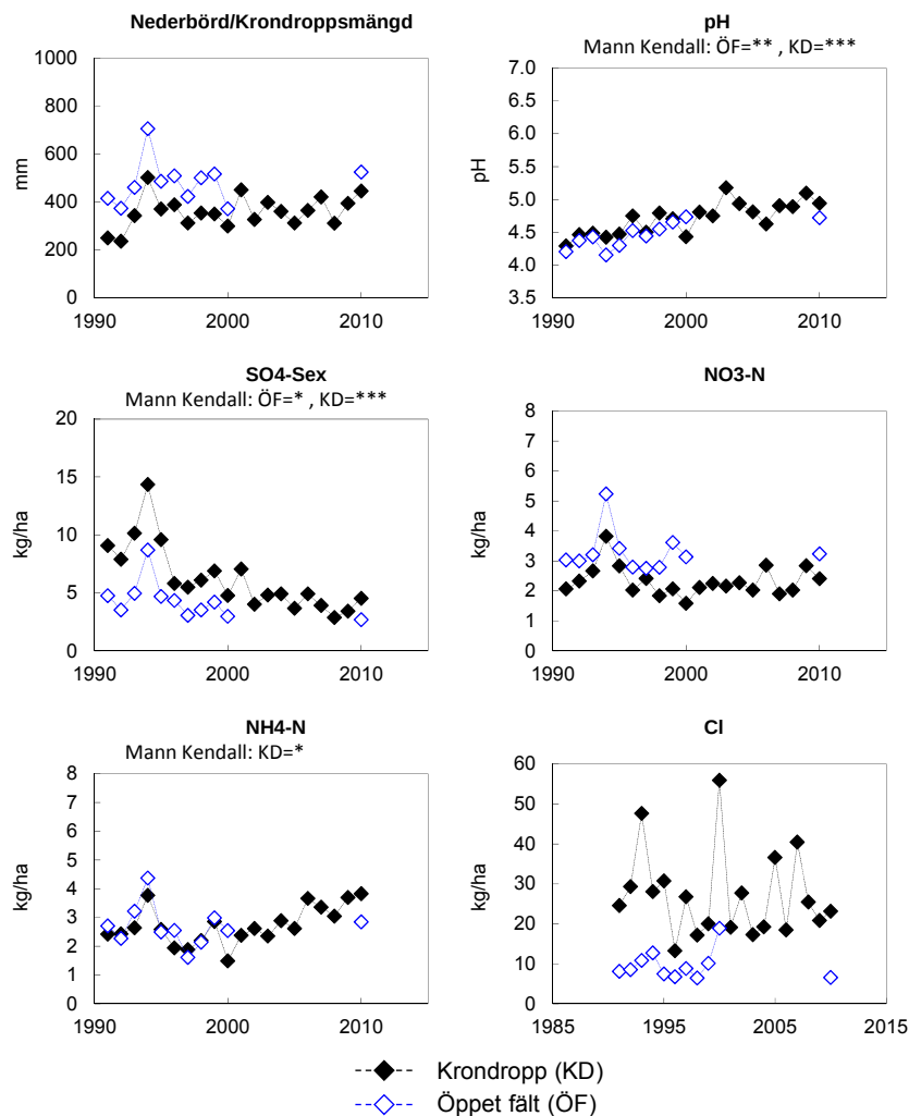
Figur 27. Årliga värden (hydrologiskt år) för depositionen i kron dropp och över öppet fält vid Ottenby, H 01 . I figuren visas uppmätt nederbörd över öppet fält samt kron droppsmängder, uttryckt som mm. pH visas för nederbörd och kron dropp. Deposition sedan mätningarna påbörjades redovisas för ett urval av ämnen: sulfatsvavel utan havssaltsbidrag (SO 4 -S ex); nitratkväve (NO 3 -N); ammoniumkväve (NH 4 -N) samt kloridjoner (Cl - ). Trendanalys har genomförts med hjälp av Mann-Kendall metodik och signifikansnivåer anges ovanför respektive diagram i de fall där signifikanta trender påvisats.
