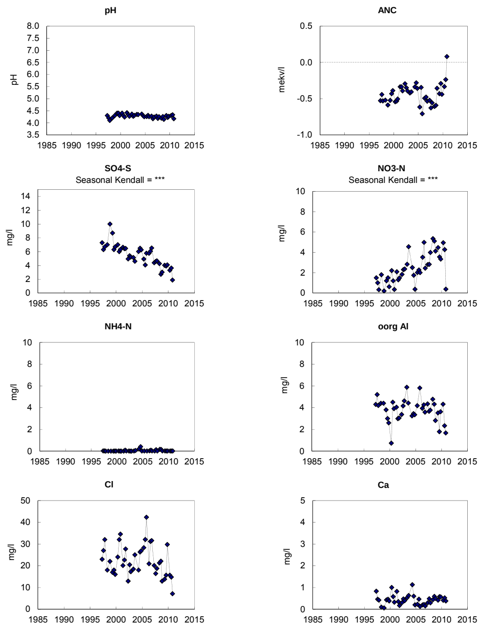
Figur 26. Markvattenkemi vid Vallåsen, N 17: pH, markvattnets syraneutraliserande förmåga (ANC), sulfatsvavel ( \text{SO}_4\text{-S} ), nitratkväve ( \text{NO}_3\text{-N} ), ammoniumkväve ( \text{NH}_4\text{-N} ) samt oorganiskt aluminium (oorg Al), kloridhalt (Cl) och kalciumhalt ( \text{Ca}^{2+} ). Saknade värden innebär oftast att marken varit för torr. Trendanalys har genomförts med hjälp av Seasonal-Kendall och signifikansnivåer anges, ovanför respektive diagram, i de fall där signifikanta trender påvisats.
