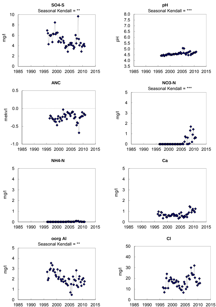
Figur 54. Markvattenkemi vid Angelstad, G 23: sulfatsvavel ( \text{SO}_4\text{-S} ), pH, markvattnets syraneutraliserande förmåga (ANC), nitratkväve ( \text{NO}_3\text{-N} ), ammoniumkväve ( \text{NH}_4\text{-N} ), kalciumhalt ( \text{Ca}^{2+} ); oorganiskt aluminium (oorg Al) samt kloridhalt (Cl). Saknade värden innebär oftast att marken varit för torr. Trendanalys har genomförts med hjälp av Seasonal-Kendall och signifikansnivåer anges, ovanför respektive diagram, i de fall där signifikanta trender påvisats.
