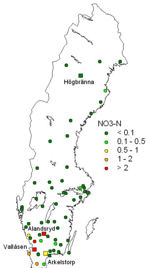
Figur 14. Nitratkväve ( \text{NO}_3\text{-N} ) i markvatten provtagen vid 50 cm djup på 60 aktiva ytor. (A). Medianvärden för perioden 2005/06 – 2007/08, tre mätningar per år per lokal. Enhet mg N/ l. Fyrkanterna i kartan visar de fyra lokalerna vars tidsserie från 1997-2008 visas i figur B och C. Tidsserierna för Högrännan (Västerbotten) och Arkelstorp (Skåne) illustrerar skillnaden mellan norra och delar av södra Sverige (B). Tidsserierna för Vallåsen och Alandsryd visar skillnaden av stormeffekten i januari 2005 som orsakade ökande nitratkoncentrationer i markvattnet.
