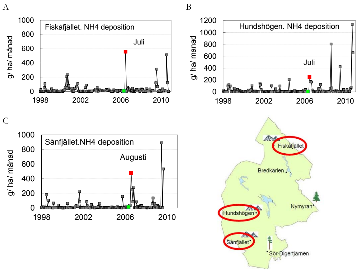
Figur 29. Månadsvisa värden för nedfall av ammonium i krondropp vid mätplatser på hög höjd (600-800 m ö.h.) i Jämtlands län, Fiskåfjellet (A), Hundshögen (B) och Sånfjället (C). Mätningarna vid Sånfjället avslutades oktober 2009. Krondroppsmätningar under gran på hög höjd bedrivs med en något annorlunda metodik jämfört med övriga Krondroppsnätet. En enda samlare finns placerad rakt under trädkronan hos vardera fem enskilda träd. Det högsta beräknade värdet markeras med rött tillsammans med en indikation för under vilken månad värdet uppträdde. Värden för maj 2006 visas med grön färgmarkering. Kartan visar Jämtlands län.
