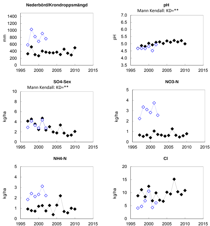
Figur 11. Årliga värden (hydrologiskt år) för deposition via kronddropp och över öppet fält vid Solltorp, E 21. I figuren visas uppmätt nederbörd över öppet fält samt kronddropsmängder, uttryckt som mm. Deposition redovisas sedan mätningarna påbörjades för ett urval av ämnen: pH; sulfatsvavel utan havssaltsbidrag (SO 4 -S ex), nitratkväve (NO 3 -N); ammoniumkväve (NH 4 -N) samt klorid (Cl). ÖF, öppet fält; KD, kronddropp. Trendanalys har genomförts med hjälp av Mann-Kendall metodik och signifikansnivåer anges ovanför respektive diagram, i de fall där signifikanta trender påvisats.
