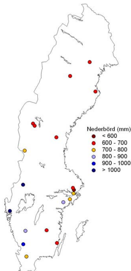
Figur 4. Nederbördsmängd under det hydrologiska året 2009/10 vid stationer inom Kron dropps nätets med mätningar över öppet fält under perioden 2000 - 2010.
