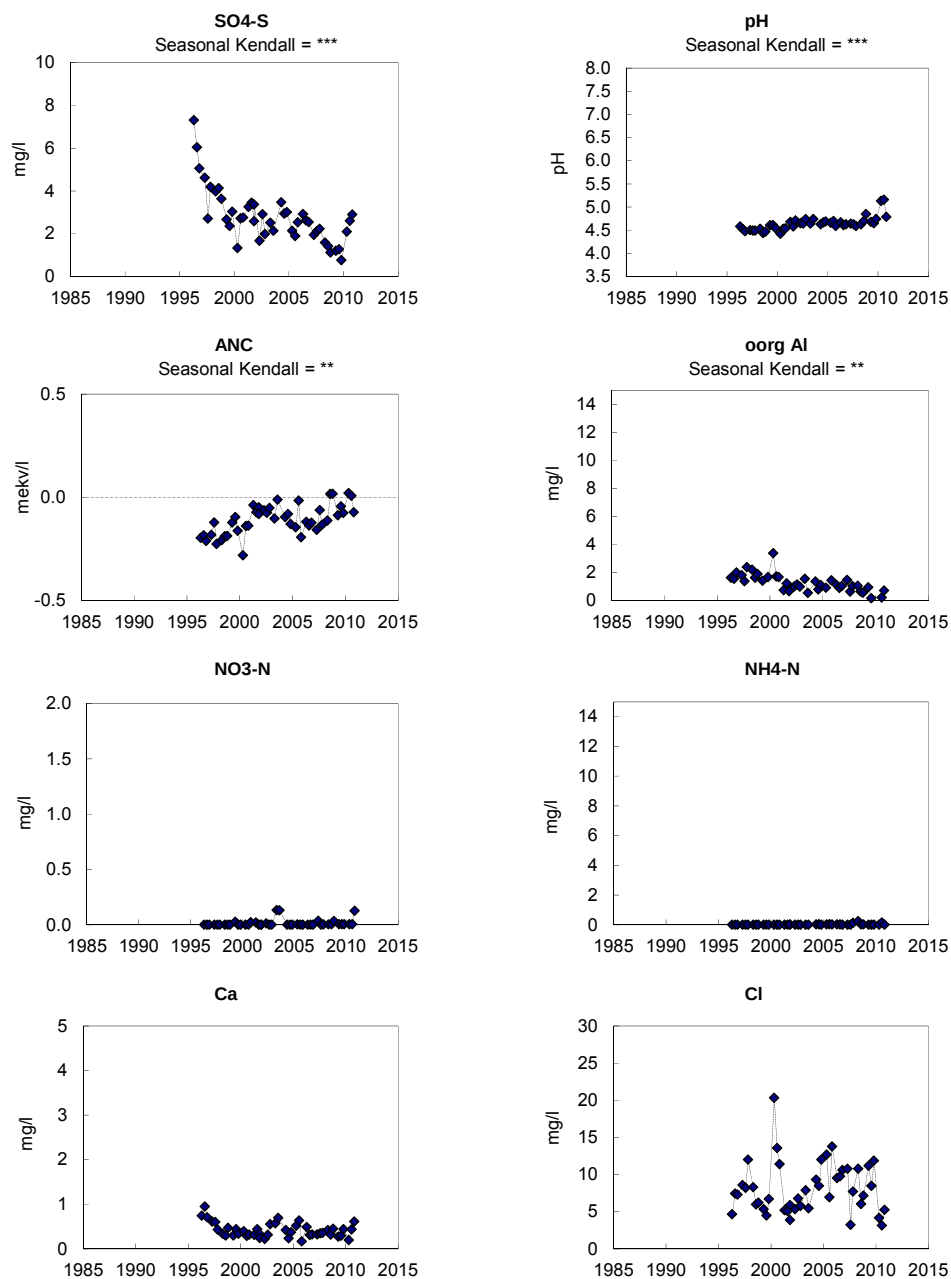
Figur 70. Markvattenkemi vid Västra Torup, L 07: sulfatsvavel ( \text{SO}_4\text{-S} ), pH, markvattnets syraneutraliserande förmåga (ANC), oorganiskt aluminium (oorg Al), nitratkväve ( \text{NO}_3\text{-N} ), ammoniumkväve ( \text{NH}_4\text{-N} ), kalciumhalt ( \text{Ca}^{2+} ) och kloridhalt (Cl). Saknade värden innebär oftast att marken varit för torr. Trend-analys har genomförts med hjälp av Seasonal-Kendall och signifikansnivåer anges, ovanför respektive diagram, i de fall där signifikanta trender påvisats.
