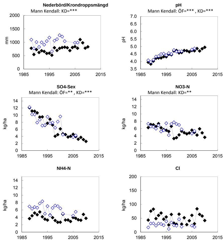
Figur 16. Årliga värden (hydrologiskt år) för depositionen via kron dropp och över öppet fält vid Söstared, N 01. I figuren visas uppmätt nederbörd över öppet fält samt kron droppsmängder, uttryckt som mm. Deposition sedan mätningarna påbörjades redovisas för ett urval av ämnen: pH; sulfatsvavel utan havssaltsbidrag (SO 4 -Sex); nitratkväve (NO 3 -N); ammoniumkväve (NH 4 -N); kloridjoner (Cl). ÖF, öppet fält; KD, kron dropp. Trendanalys har genomförts med hjälp av Mann-Kendall-analys och signifikansnivåer anges, ovanför respektive diagram, i de fall där signifikanta trender påvisats.
