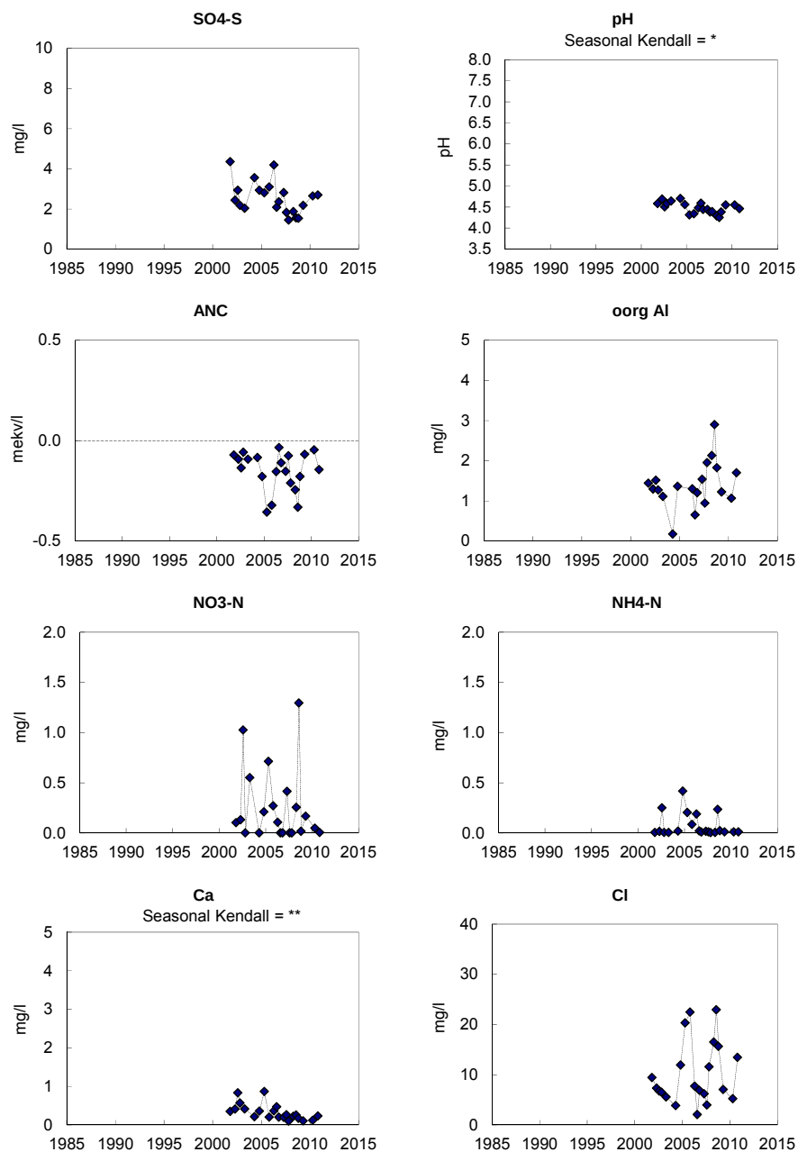
Figur 75. Markvattenkemi vid Maryd, L 15 : sulfatsvavel ( \text{SO}_4\text{-S} ), pH, markvattnets syraneutraliserande förmåga (ANC), oorganiskt aluminium (oorg Al), nitratkväve ( \text{NO}_3\text{-N} ), ammoniumkväve ( \text{NH}_4\text{-N} ), kalciumhalt ( \text{Ca}^{2+} ) och kloridhalt ( \text{Cl}^- ). Saknade värden innebär oftast att marken varit för torr. Trendanalys har genomförts med hjälp av Seasonal-Kendall och signifikansnivåer anges, ovanför respektive diagram, i de fall där signifikanta trender påvisats.
