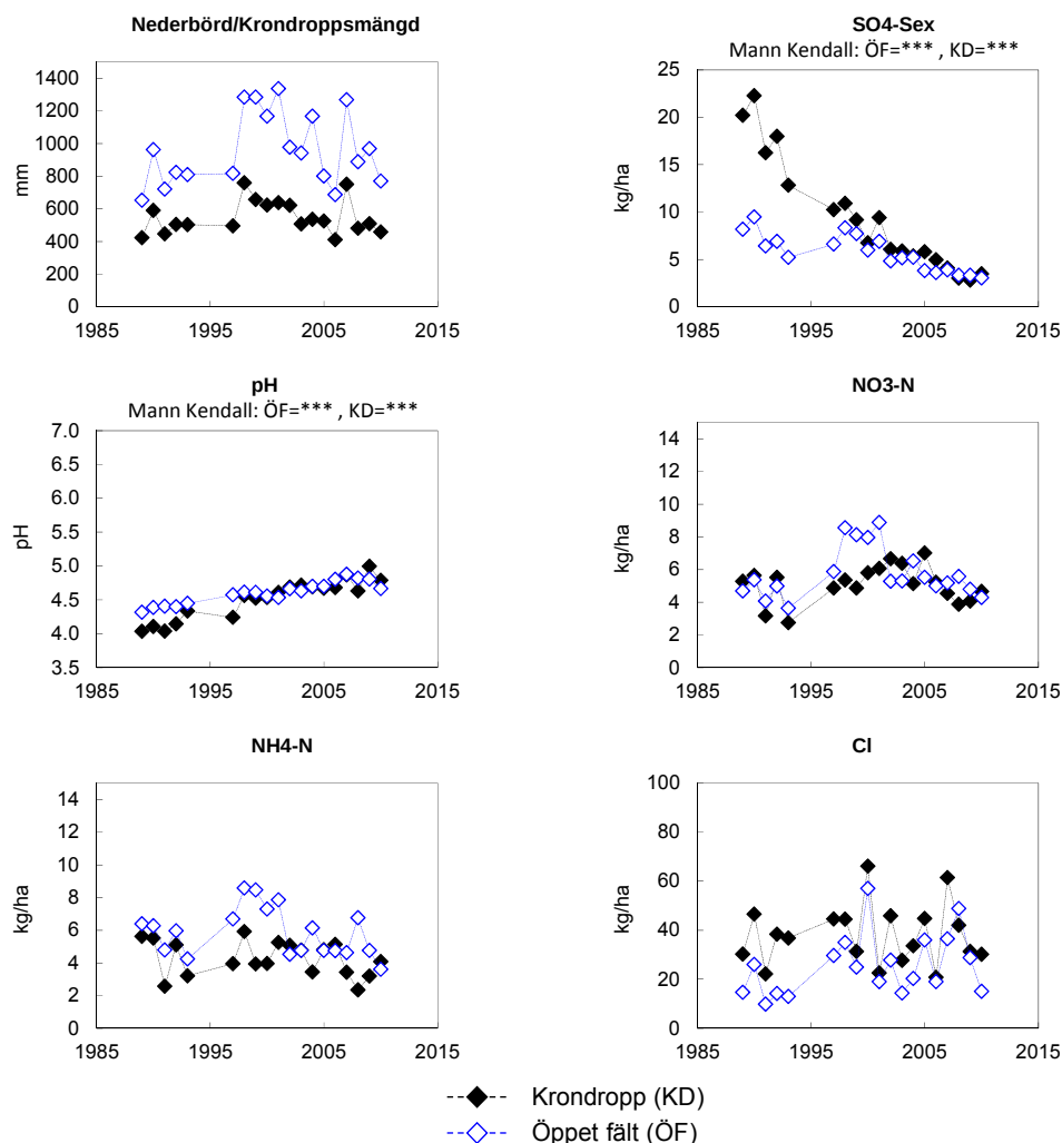
Figur 69. Årliga värden (hydrologiskt år) för depositionen via krondropp och över öppet fält vid Västra Torup, L 07 . I figuren visas uppmätt nederbörd över öppet fält samt krondroppsmängder, uttryckt som mm. Deposition sedan mätningarna påbörjades redovisas för ett urval av ämnen: sulfatsvavel utan havssaltsbidrag (SO 4 -S ex); pH, nitratkväve (NO 3 -N); ammoniumkväve (NH 4 -N); kloridjoner (Cl - ). ÖF, öppet fält; KD, krondropp. Trendanalys har genomförts med hjälp av Mann-Kendall analys och signifikansnivåer anges ovanför respektive diagram då signifikanta trender påvisats. Observera att krondroppsmätningarna från 1996 och framåt utfördes på en annan yta inom beståndet än tidigare.
