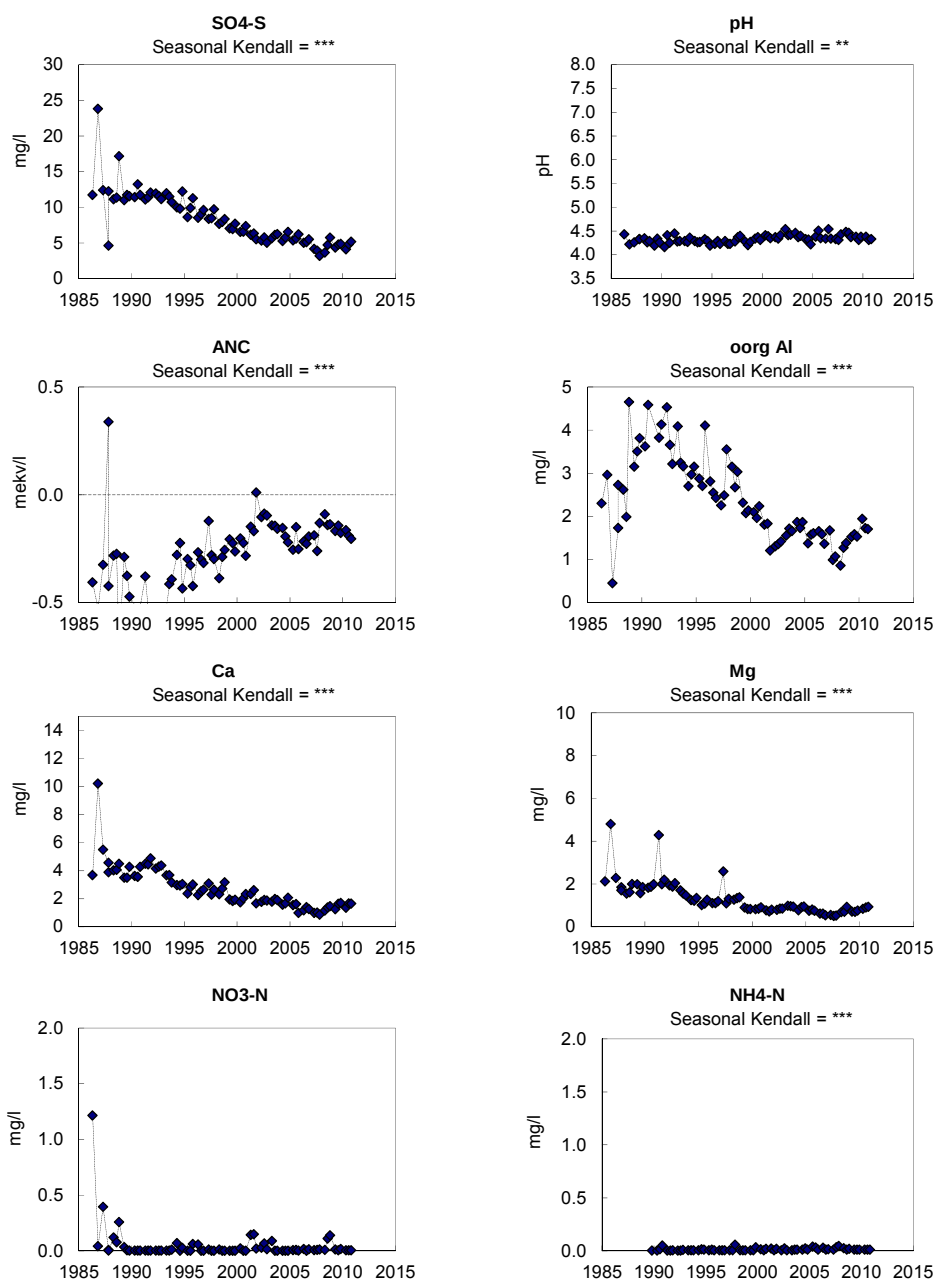
Figur 41. Markvattenkemi vid Ryssberget, K 07 . Sulfatsvavel ( \text{SO}_4\text{-S} ); pH; markvattnets syraneutraliserande förmåga (ANC); oorganiskt aluminium (oorg Al); kalciumhalt ( \text{Ca}^{2+} ); magnesium ( \text{Mg}^{2+} ); nitratkväve ( \text{NO}_3\text{-N} ) samt ammoniumkväve ( \text{NH}_4\text{-N} ). Saknade värden innebär oftast att marken varit för torr. Trendanalys har genomförts med hjälp av Seasonal-Kendall metodik och signifikansnivåer anges, ovanför respektive diagram, i de fall där signifikanta trender påvisats.
