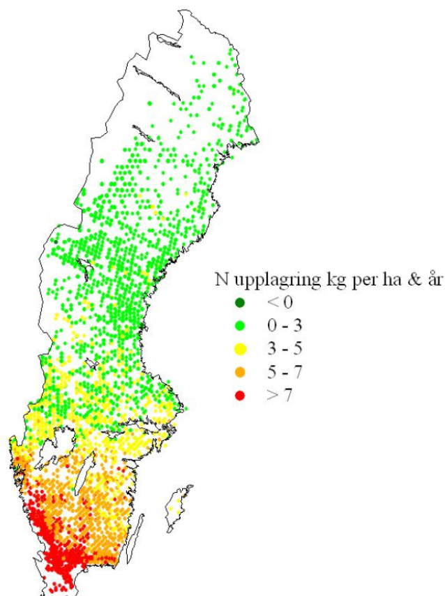
Figur 22. Kväveackumulering i granskog vid ett skogsbrukscenario baserat på enbart stamvedsuttag, baserat på kvävenedfall nedfall från åren 2003-2005 (medelvärde). (Akselsson m. fl., 2010).
