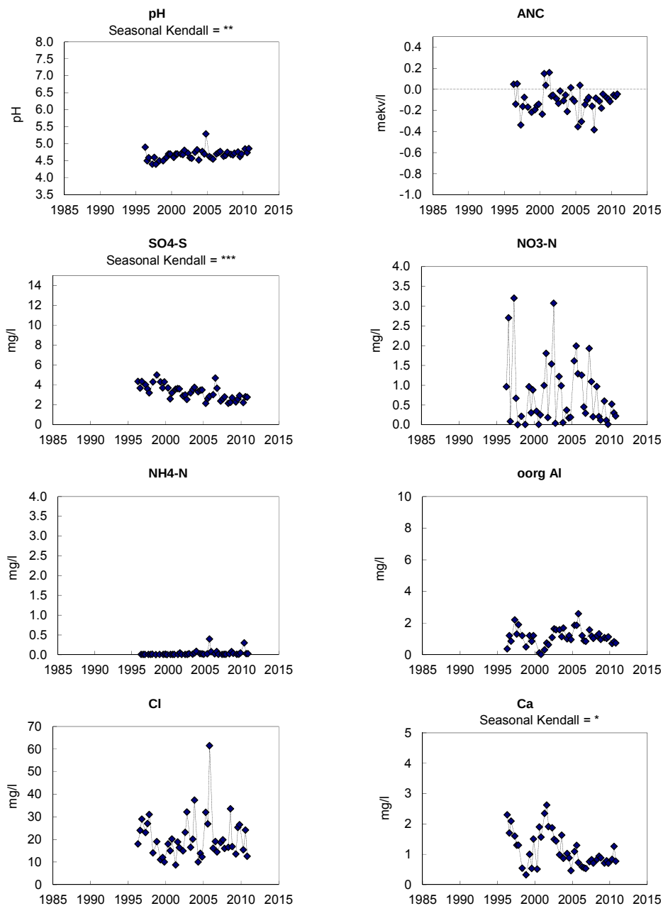
Figur 24. Markvattenkemi vid Djupeåsen, N 14: pH, markvattnets syraneutraliserande förmåga (ANC), sulfatsvavel ( \text{SO}_4\text{-S} ), nitratkväve ( \text{NO}_3\text{-N} ), ammoniumkväve ( \text{NH}_4\text{-N} ), oorganiskt aluminium (oorg Al), kloridhalt ( \text{Cl}^- ) och kalciumhalt ( \text{Ca}^{2+} ). Saknade värden innebär oftast att marken varit för torr. Trendanalys har genomförts med hjälp av Seasonal-Kendall och signifikansnivåer anges, ovanför respektive diagram, i de fall där signifikanta trender påvisats.
