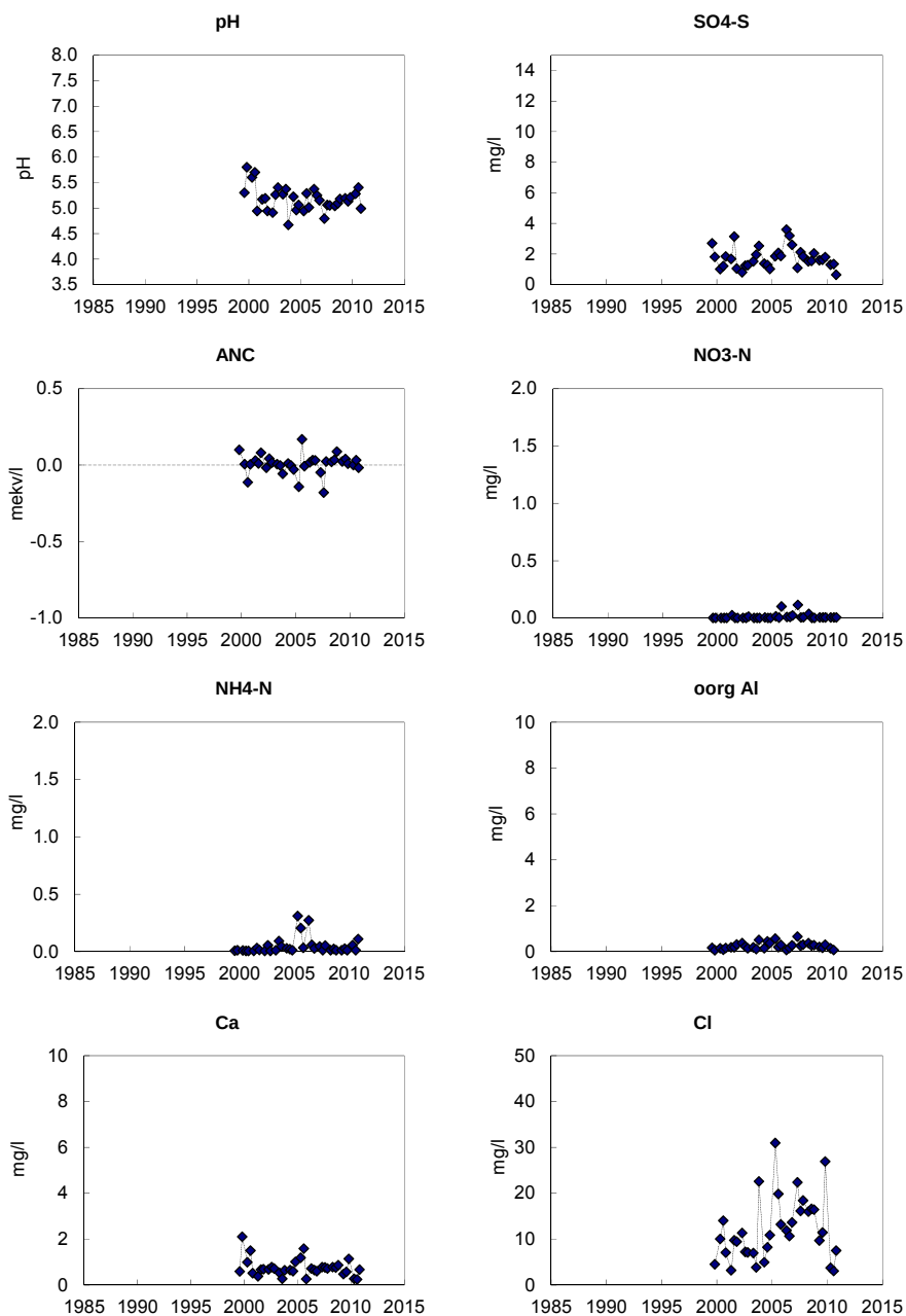
Figur 17. Markvattenkemi vid Söstared, N 01-B: pH, sulfatsvavel (SO 4 -S), markvattnets syraneutraliserande förmåga (ANC), nitratkväve (NO 3 -N), ammoniumkväve (NH 4 -N), oorganiskt aluminium (oorg Al), kalciumhalt (Ca 2+ ) och kloridhalt (Cl). Saknade värden innebär oftast att marken varit för torr. Trendanalys har genomförts med hjälp av Seasonal-Kendall och signifikansnivåer anges, ovanför respektive diagram, i de fall där signifikanta trender påvisats.
