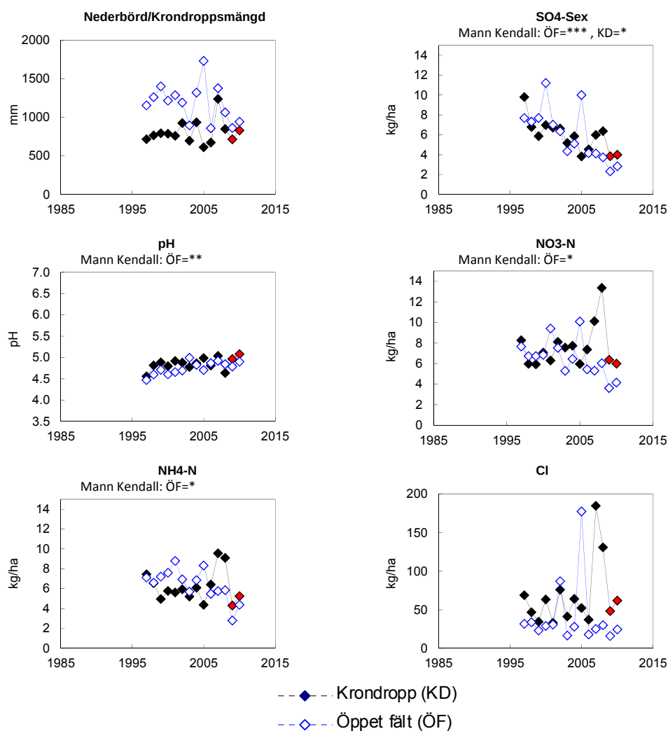
Figur 20. Årliga värden (hydrologiskt år) för depositionen via kronddropp och över öppet fält vid Timrilt, N 13. I figuren visas uppmätt nederbörd över öppet fält samt kronddroppsmängder, uttryckt som mm. Deposition sedan mätningarna påbörjades redovisas för ett urval av ämnen: sulfatsvavel utan havssaltsbidrag ( \text{SO}_4\text{-S ex} ); pH; nitratkväve ( \text{NO}_3\text{-N} ); ammoniumkväve ( \text{NH}_4\text{-N} ); kloridjoner (Cl). ÖF, öppet fält; KD, kronddropp. När det gäller kronddroppsmätningarna så flyttades de i oktober 2008 varför senare mätningar anges med en röd symbol. Trendanalys har genomförts med hjälp av Mann-Kendall-analys och signifikansnivåer anges, ovanför respektive diagram, i de fall där signifikanta trender påvisats. I de fall där statistiskt signifikanta trender erhålls i kronddropp gäller de enbart mätningar vid den gamla ytan.
