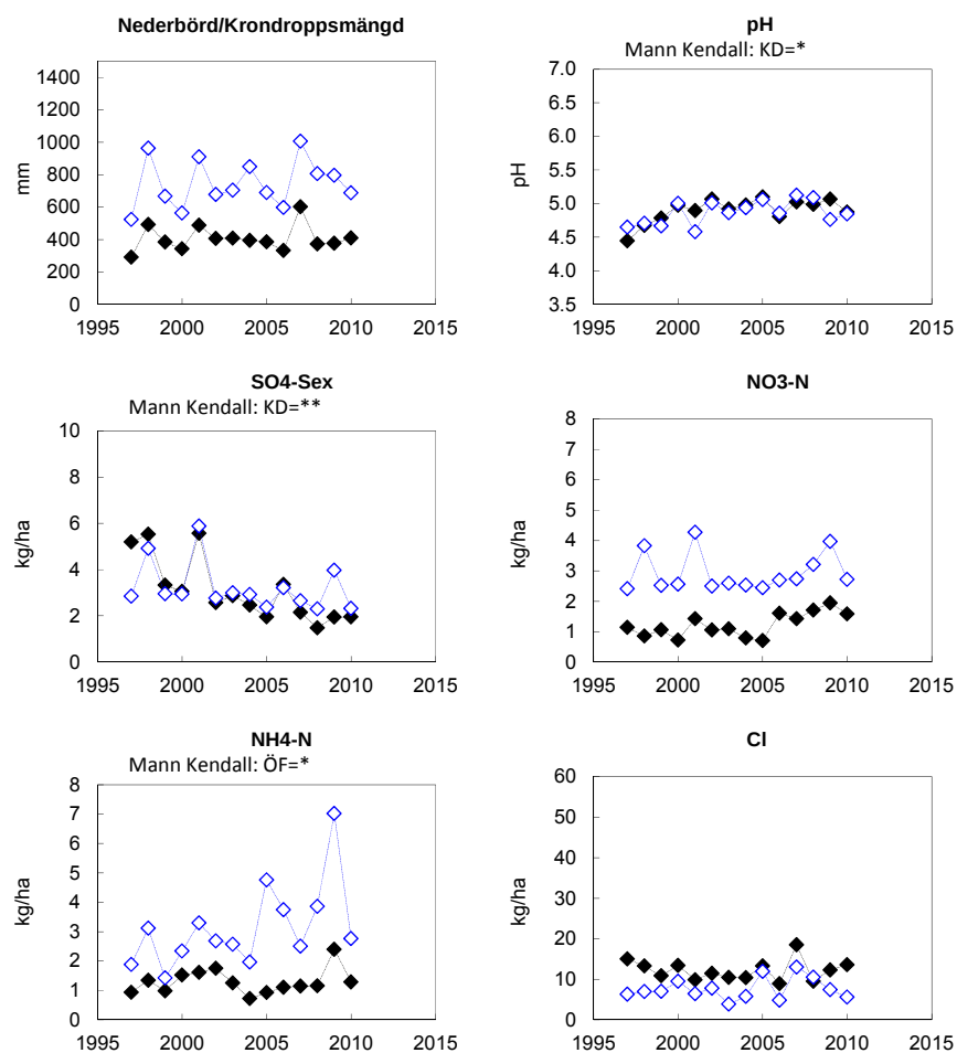
Figur 8. Årliga värden (hydrologiskt år) för depositionen via krondropp och över öppet fält vid Fagerhult, F23 . I figuren visas uppmätt nederbörd över öppet fält samt krondroppsmängder, uttryckt som mm. Deposition sedan mätningarna påbörjades redovisas för ett urval av ämnen: pH; sulfatsvavel utan havssaltsbidrag (SO 4 -S ex), nitratkväve (NO 3 -N); ammoniumkväve (NH 4 -N); kloridjoner (Cl). ÖF, öppet fält; KD, krondropp. Trendanalys har genomförts med hjälp av Mann-Kendall analys och signifikansnivåer anges, ovanför respektive diagram, i de fall där signifikanta trender påvisats.
