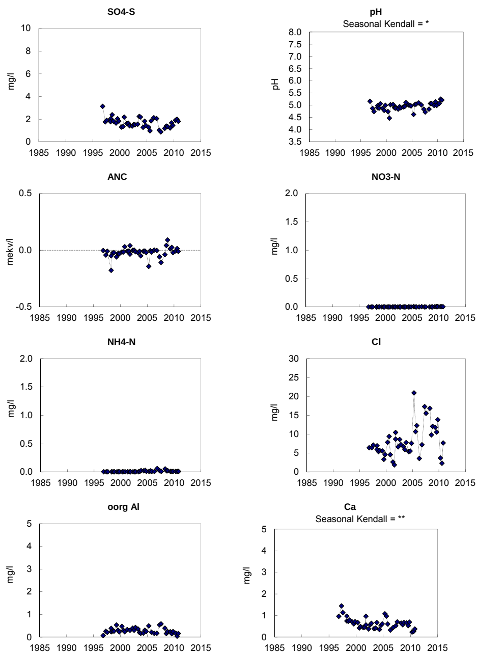
Figur 56. Markvattenkemi vid Åboland, O 01: sulfatsvavel ( \text{SO}_4\text{-S} ), pH, markvattnets syraneutraliserande förmåga (ANC), nitratkväve ( \text{NO}_3\text{-N} ), ammoniumkväve ( \text{NH}_4\text{-N} ), kloridhalt ( \text{Cl} ); oorganiskt aluminium (oorg Al) samt kalciumhalt ( \text{Ca}^{2+} ). Saknade värden innebär oftast att marken varit för torr. Trendanalys har genomförts med hjälp av Seasonal-Kendall och signifikansnivåer anges, ovanför respektive diagram, i de fall där signifikanta trender påvisats.
