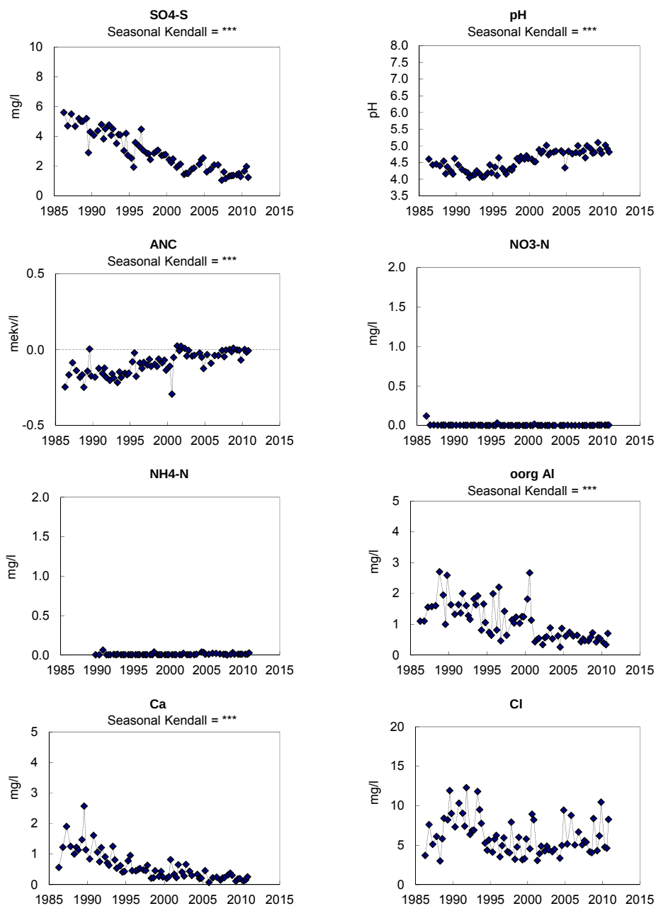
Figur 39. Markvattenkemi vid Hjärtsjömåla, K 03. Sulfatsvavel ( \text{SO}_4\text{-S} ); pH; markvattnets syraneutraliserande förmåga (ANC); nitratkväve ( \text{NO}_3\text{-N} ); ammoniumkväve ( \text{NH}_4\text{-N} ); oorganiskt aluminium (oorg Al); kalciumhalt ( \text{Ca}^{2+} ); kloridhalt (Cl). Saknade värden innebär oftast att marken varit för torr. Trendanalys har genomförts med hjälp av Seasonal-Kendall metodik och signifikansnivåer anges, ovanför respektive diagram, i de fall där signifikanta trender påvisats.
