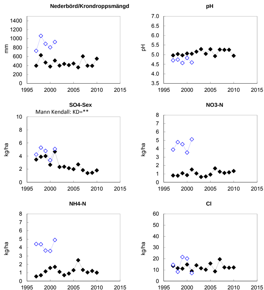
Figur 6. Årliga värden (hydrologiskt år) för depositionen via krondropp och över öppet fält vid Bordsjö, F 22 . I figuren visas uppmätt nederbörd över öppet fält samt kron-droppsmängder, uttryckt som mm. Deposition sedan mätningarna påbörjades redovisas för ett urval av ämnen: pH; sulfatsvavel utan havssaltsbidrag (SO 4 -S ex), nitratkväve (NO 3 -N); ammoniumkväve (NH 4 -N); kloridjoner (Cl). ÖF, öppet fält; KD, krondropp. Trendanalys har genomförts med hjälp av Mann-Kendall analys och signifikansnivåer anges, ovanför respektive diagram, i de fall där signifikanta trender påvisats.
