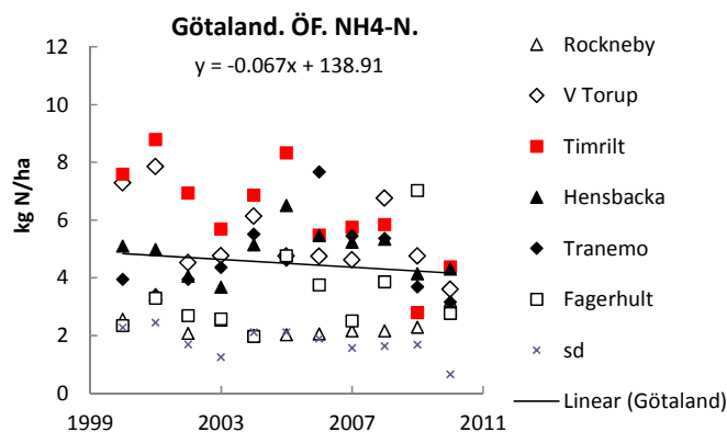
Figur 20. Tidsutvecklingen för nedfallet av nitratkväve (NO 3 -N) och ammoniumkväve (NH 4 -N) över öppet fält (ÖF) vid olika platser i Götaland under 2000-talet. Nedfall av NO 3 -N (A), Nedfall av NH 4 -N (B). Linjär regression för de årliga medelvärdena baserat på alla platser inom områden visas tillsammans med den årliga standardavvikelsen. Symboler för platser med statistiskt säkerställda förändringar över tid visas med rött.
