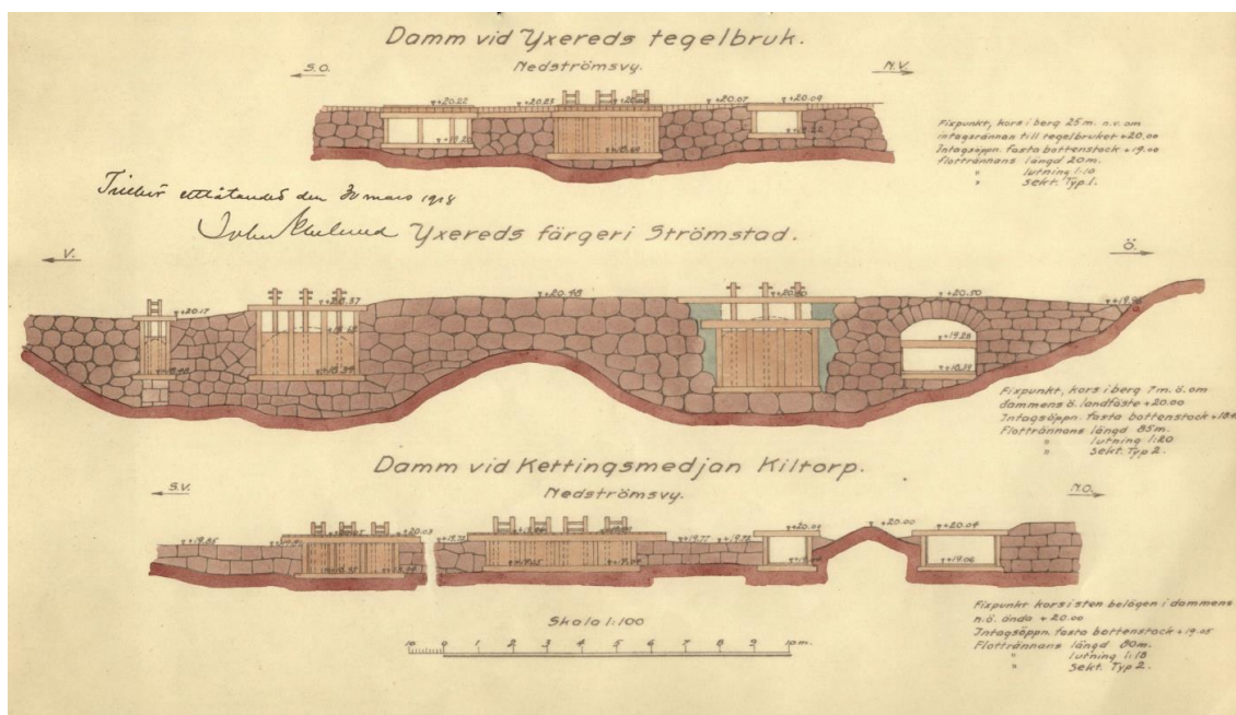
Uppmätning av dammar vid Yxered och Kiltorp från år 1918. Riksarkivet, Väg- och vattenbyggnadsstyrelsens arkiv, Östra distriktet. Foto: Riksarkivet
