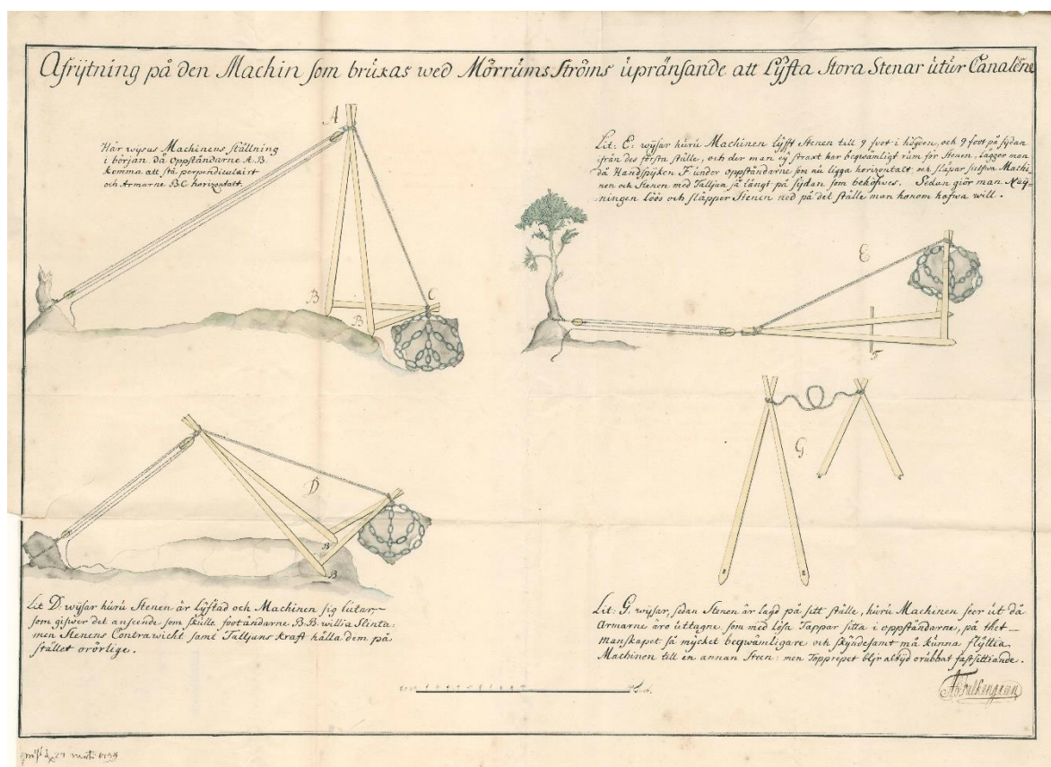
Avrättning av en maskin som använts för stenrensning i Mörrumsån. Avrättningen är utförd 1734. Riksarkivet. Kollegier med flera landshövdingars, hovrätters och konsistoriers skrivelser till Kungl. Maj:t. Skrivelser till amiralitetskollegiet. Foto: Riksarkivet.
