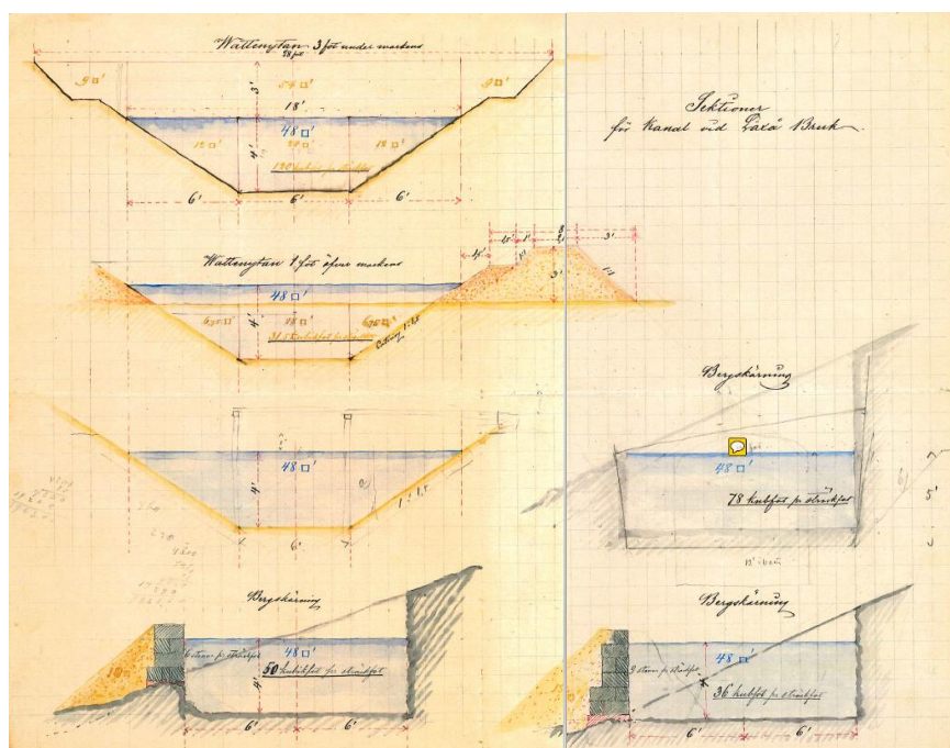
Projekt till kanal vid sulfittfabrik vid Laxå bruk år 1888. (Ritningen är scannad i två delar.) ArkivCentrum Örebro, Laxå bruksarkiv.
