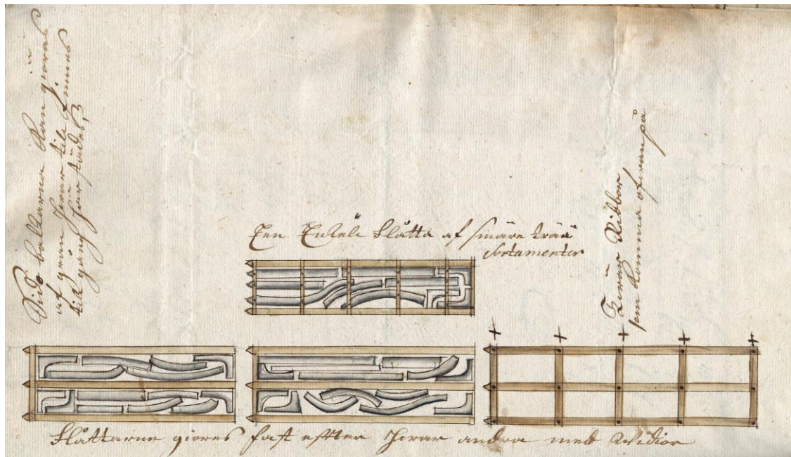
Principritning över furuflotte för transport av ekstockar, upprättad år 1735. Riksarkivet, Amiralitetskollegiet. Foto: Riksarkivet.
