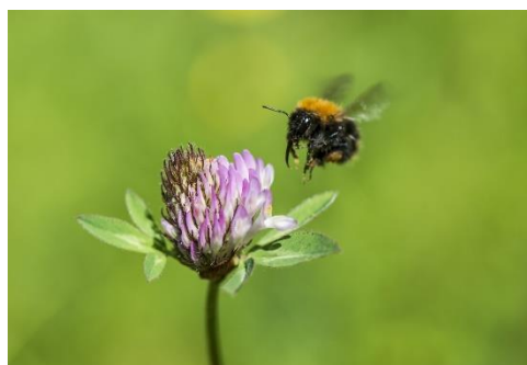
Figur 13. Pollinerande insekters livscyklar kommer i obalans i ett förändrat klimat. Foto: Länsstyrelsen.
