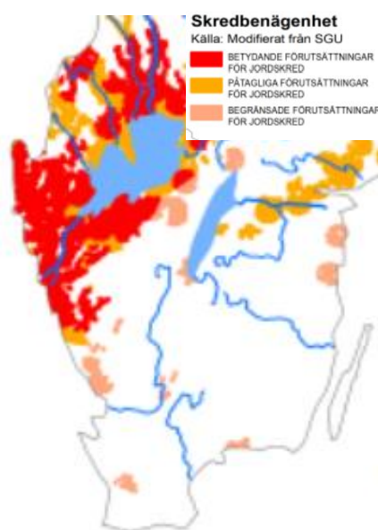
Figur 6. Risköversikt för benägenhet för jordskred i södra Sverige. (SGI och MSB, 2021)
