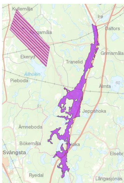
Figur 7: Exempel på två olika geologiska formationer med god grundvattentillgång.
