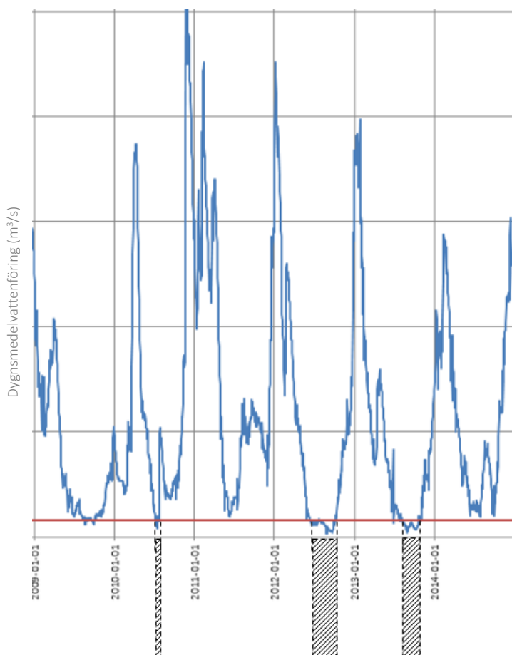
Figur 15: Dygnsmedelföringens variation i ett vattendrag 2009–2015. Röd linje utgör stoppgräns för vattenuttag (9,99 procent sänkning av MLQ). Rastrerade fält markerar tidsperioder när vattenföringen understiger stoppgränsen.
