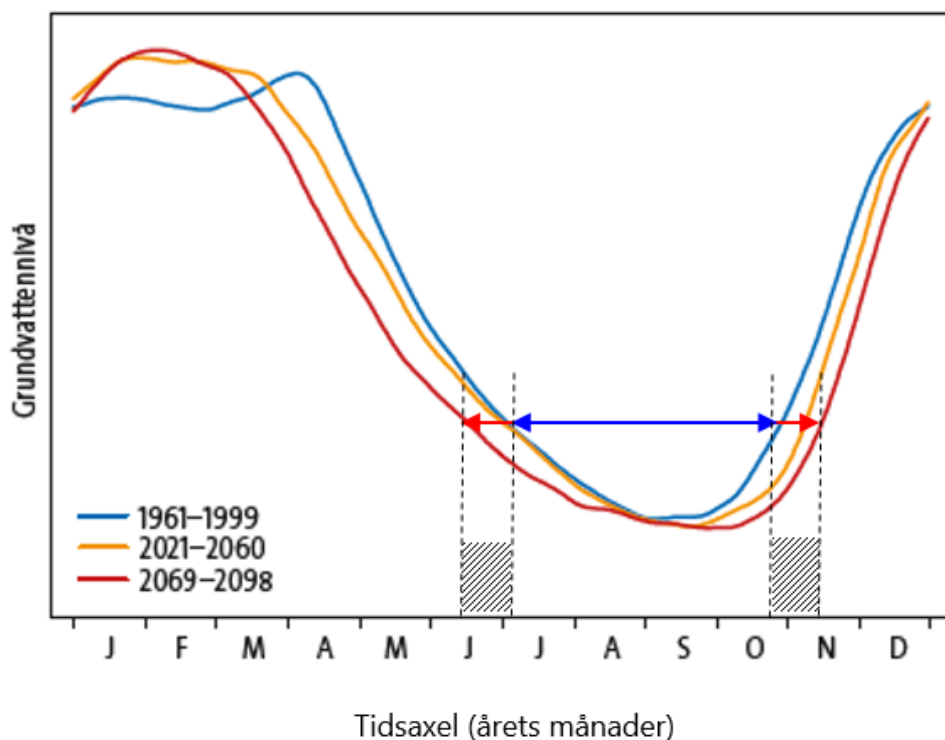
Figur 11: Kurvorna visar årstidsvariation i grundvattennivå för referensperioden 1961–1990 och för perioderna 2021–2060 och 2069–2098 (dygnsmedelvärden för ett snabbreagerande grundvattenmagasin i sydöstra Sverige). Rastrerat område visar hur perioden med låg grundvattentillgång förlängs mellan referensperioden och 2069–2098. Bearbetad figur från SOU 2015:51.
