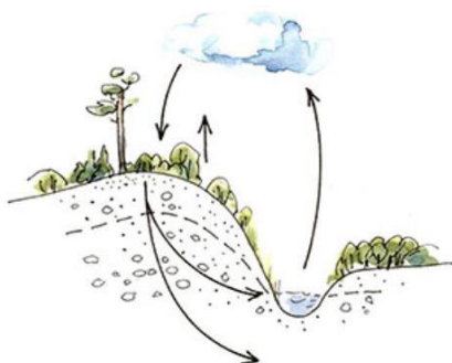
Figur 6: Den streckade linjen illustrerar grundvattenytan. Under den nivån är alla porer och håligheter i marken fyllda med vatten – grundvatten. Grundvattnet utgör en del i vattnets naturliga kretslopp.
