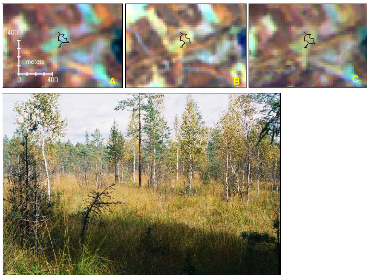
Figur 64. En av de tre ytorna inom "ökad biomassa/igenväxning 3/2-kvoten" som inte kunnat verifieras som förändrad vid utvärderingen. Orsaken är troligen att blååteln och porsen i fältskiktet inte var fullt utvecklade vid registreringsstillfället 1986-06-11 jämfört med den senare tidpunkten 2001-08-15. A. 1986-06-11 B. 2001-08-15 C. 1985-09-12 för jämförelse. D. Markfoto taget i september 2003 av Thomas Rafstedt.
