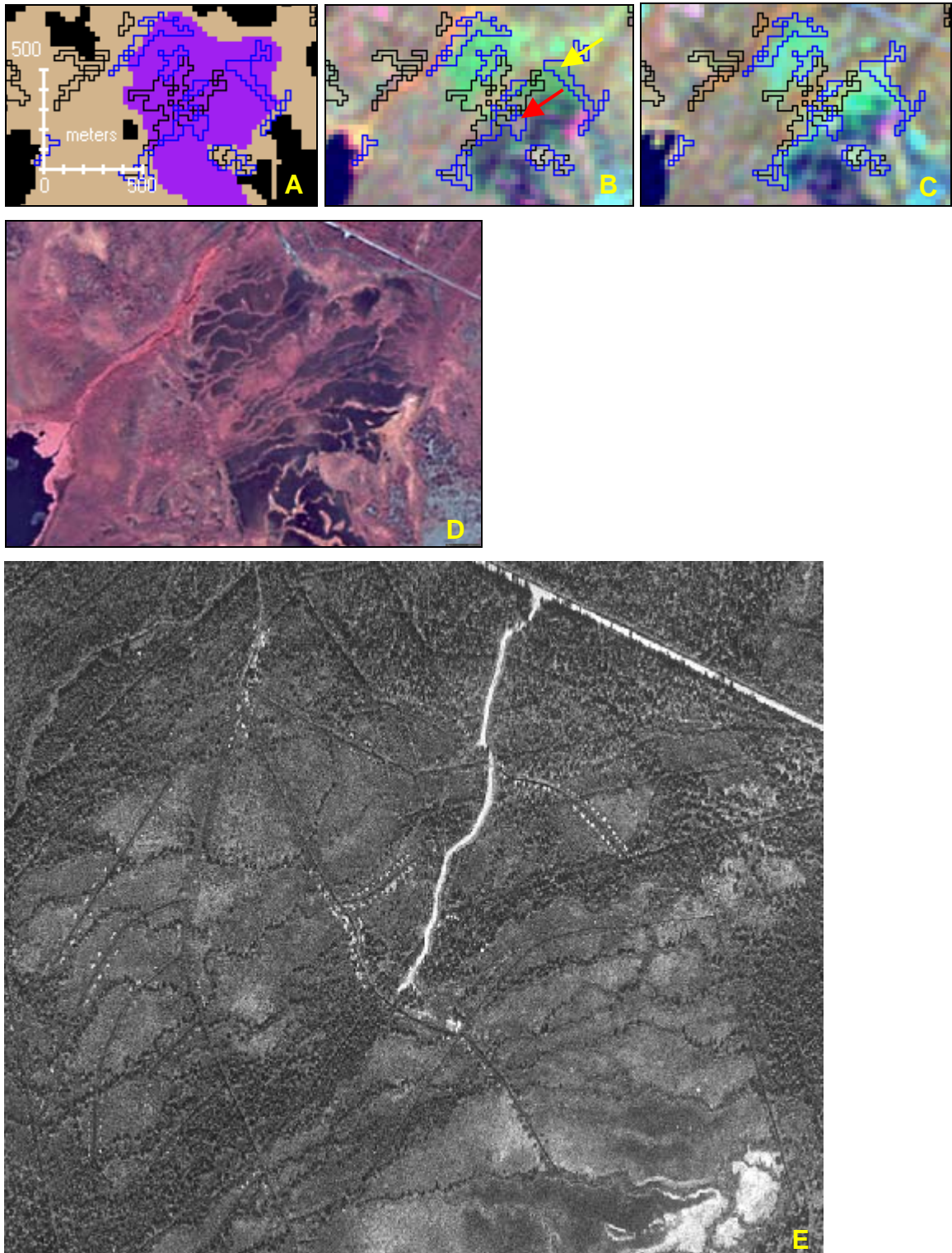
Figur 72. Fd strängblandmyr med uppslag av tall och björk i flarkarna. Området är kraftigt dikat. Dikningen utförd för ca 10-15 år sedan. Del av VMI klass 1-objekt. A. Myrmasker från Vägkartan, beige = öppen brunmyr, lila = öppen blåmyr. svarta polygoner = ökad biomassa/igenväxning, blå polygoner = förändrat botten/fältskikt. B. 1987-08-10. C. 2000-07-29. D. IR-färgflygbild från 1979-07-16. E. Ortofoto från 1997. Gul pil visar plats för markbild i figur 73. Röd pil visar plats för markbilder i figur 74.
