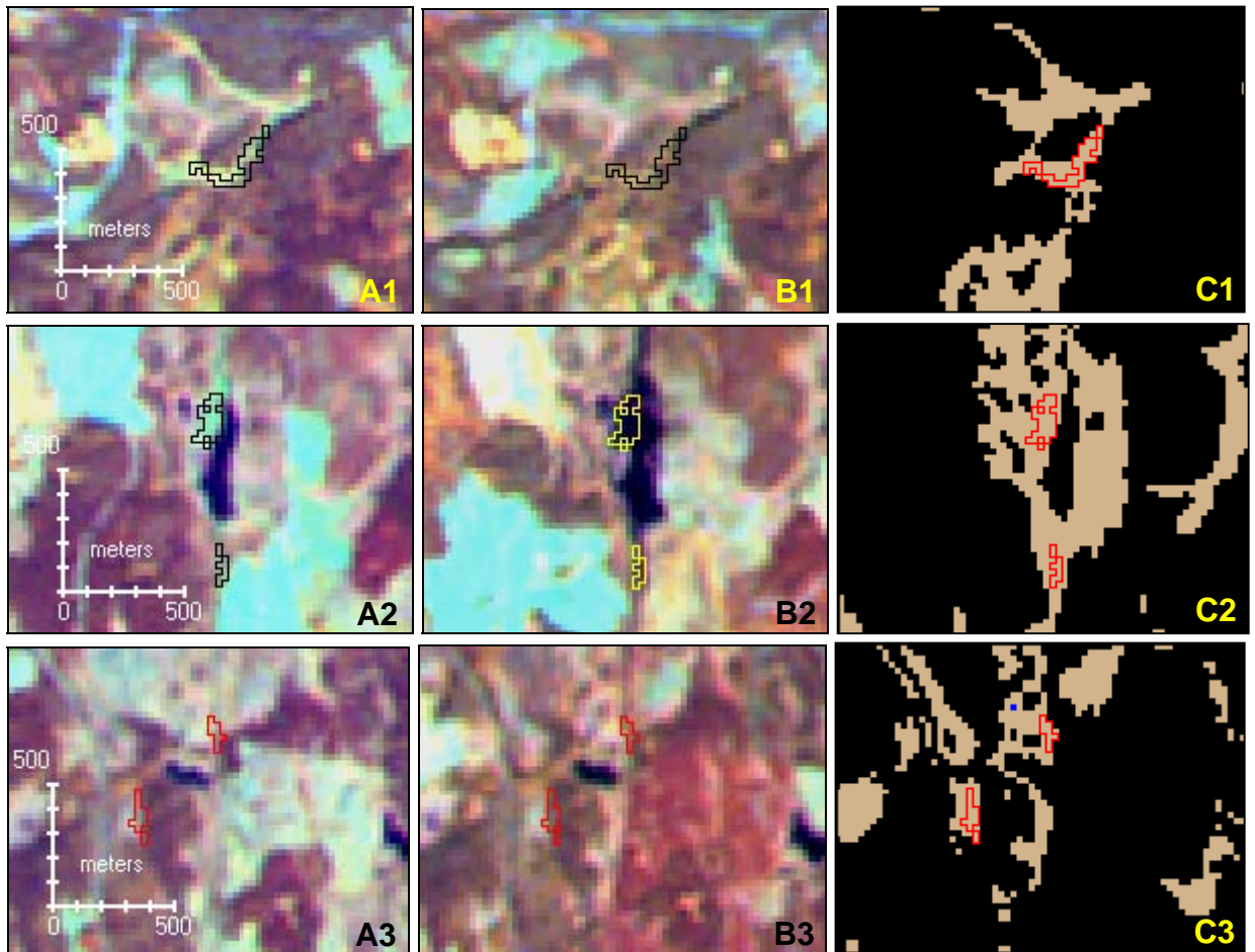
Figur 50. Exempel på förändringar som fallit ut inom delresultatet "ökad biomassa/igenväxning" inom rött scenpar. 1. Igenväxning. 2. Effekt av mycket hög nederbörd sommaren 2000 (se avsnitt 3. 3.1.5). Svårbedömt om förändringarna är kanteffekter. A. 1989-08-22 B. 2000-07-28 C. Myrmaskerna från terrängkartan, beige = öppen brunmyr, lila = öppen blåmyr.
