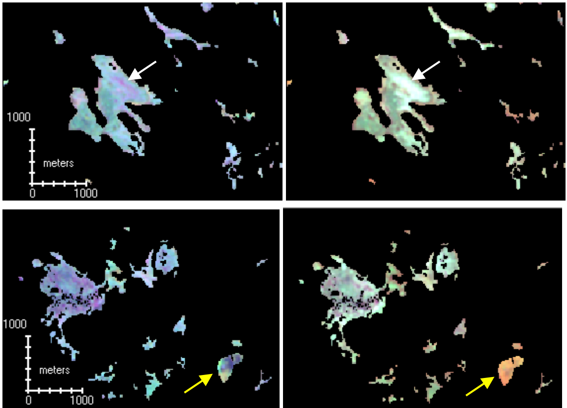
Figur 13. Exempel på skillnader mellan de två registreringstillfällena, 1986-06-13 (bilder till vänster) och 2001-07-07 (bilder till höger) inom blått scenpar, som både beror på fenologiska skillnader (gul pil, vegetationens utveckling) och skillnader i nederbördsförhållanden (vit pil).
