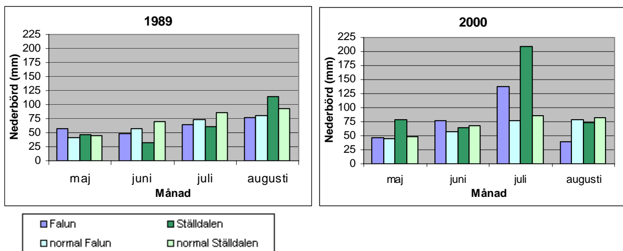
Figur 10. Månadsnederbörd för Falun och Ställdalen meteorologiska stationer för maj - augusti de år som använda satellitbilder registrerats (1989-08-22 respektive 2000-07-28).
