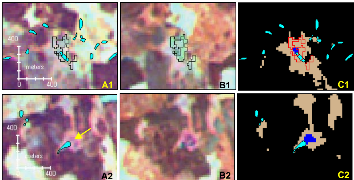
Figur 51. A1-ytorna visar förändringar som fallit ut inom delresultatet "förändringar av bottenskikt/fältskikt" inom rött scenpar som kan kopplas till kalkning (ljusblå polygoner). A2-serien visar en Sphagnum-dominerad myr (gul pil) som inte tycks ha påverkats i någon större omfattning av kalkningen. A. 1989-08-22 B. 2000-07-28 C. Myrmaskerna från terrängkartan, beige = öppen brunmyr, blått = öppen blåmyr.
