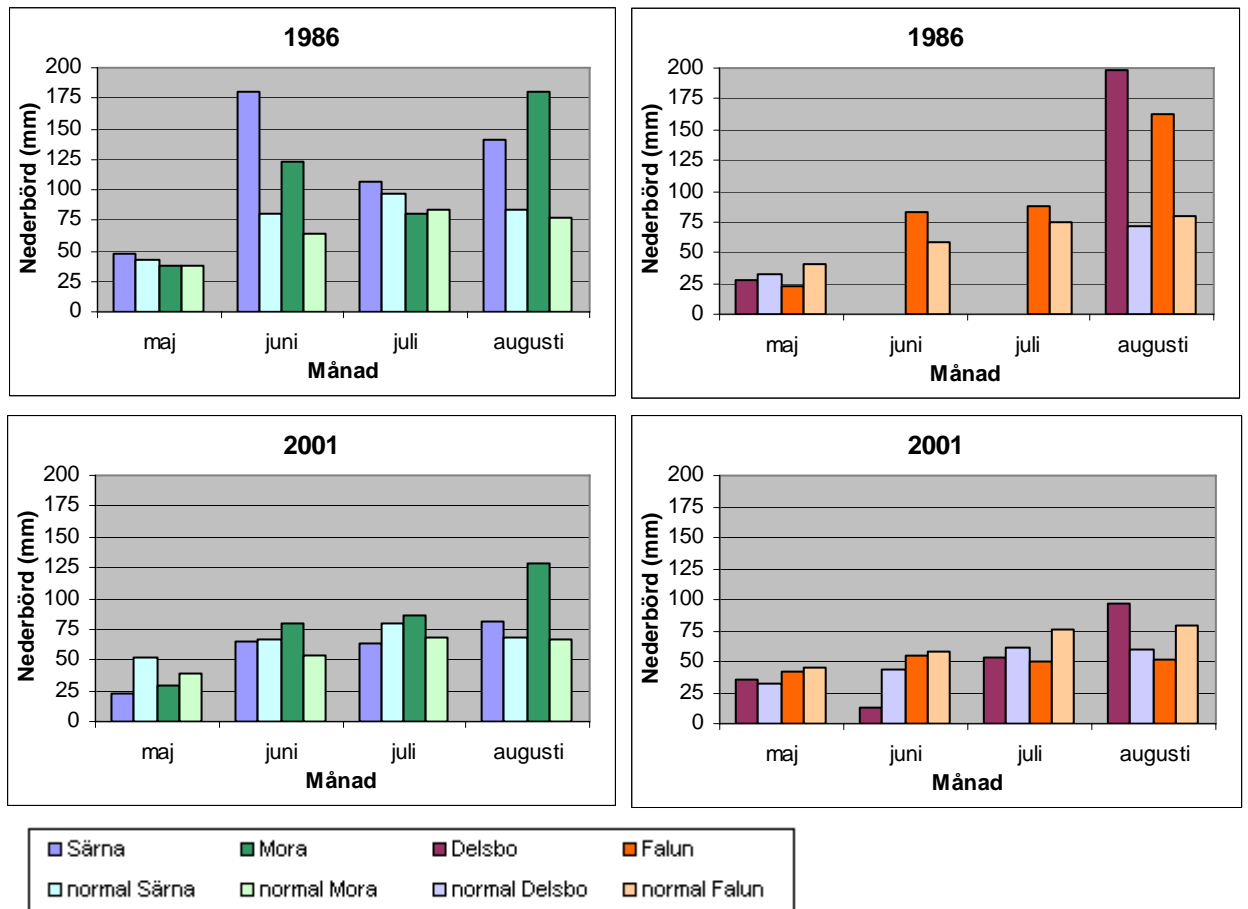
Figur 8. Månadsnederbörd för Särna, Mora, Delsbo och Falun meteorologiska stationer för maj - augusti de år som använde satellitbilder registrerats (1986-06-11 respektive 2001-08-15).
