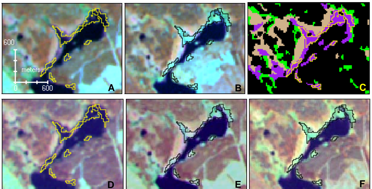
Figur 41. Exempel på förändringar som fallit ut som "förändrat bottenstikt/fältskikt" inom myrar som varit mycket blöta 86-06-11 (typ lösbottnar, sumpkärr eller andra blöta våtmarker) inom orange scenpar, 200-500 m.ö.h. A. 1986-06-11 B. 2001-08-15 C. Myrmaskerna från terrängkartan, grönt = skogklädd myr, beige = öppen brunmyr, lila = öppen blåmyr D. 1985-09-12 E. 1992-05-19 F. 1997-08-21.
