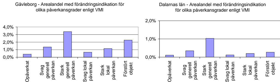
Figur 80. Diagram över förändringsindikation i olika påverkanssklasser i Våtmarksinventeringen, VMI.
