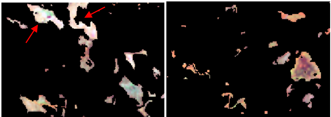
Figur 16. Områdena i mellersta och nedersta bildparen i figur 15 i satellitbild från 2001-07-07, vilken försiggick av extremt torrt väder. Jämför t ex de Sphagnum-dominerade myrarna i den vänstra bilden med desamma 1986 respektive 2001 i augusti (röda pilar).
