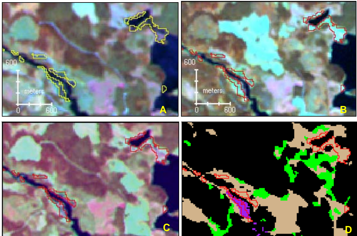
Figur 40. Exempel på förändringar som fallit ut som "förändrat bottenstikt/fältskikt" inom myrar som varit mycket blöta 86-06-11 (typ lösbottnar, sumpkärr eller andra blöta våtmarker) inom orange scenpar, 200-500 m.ö.h. A. 1986-06-11 B. 2001-08-15 C. 1992-05-19 D. Myrmaskerna från terrängkartan, grönt = skogklädd myr, beige = öppen brunmyr, lila = öppen blåmyr.
