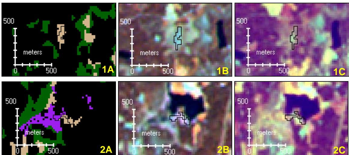
Figur 66. Ytterligare exempel på igenväxning inom kartbladet 6E SV. 1. Dikad öppet kärr som idag inte längre är att betrakta som myrsmark. 2. Fastmattekärr som fått ett förtätat uppslag av 1 meters björka. A. Myrmasker från fastighets-kartan. grönt = skogklädd myr, beige = öppen brunmyr, öppen blåmyr. B. 1985-06-01 C. 2002-07-10. Markbilder visas i figur 67.
