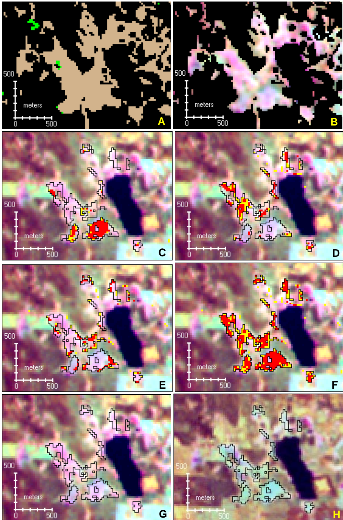
Figur 25. Förändring av bottenskiktet mellan 1986 och 2001 norr om Siljan, Dalarna. Exempel på hur ett samlat förändringsresultat skapas genom hopslagning av olika delmängder. A. Myrmark B. Öppen myr i satellitbild från 1986-06-18. C-E. Delresultat, rött=säker förändring, gul= potentiell förändring. F. Hoplagt, ej generaliserat resultat. G. Generaliserat slutresultat (svart polygon) lagt på satellitbild från 1986-06-18. D. Generaliserat slutresultat (svart polygon) lagt på satellitbild från 2001-08-15
