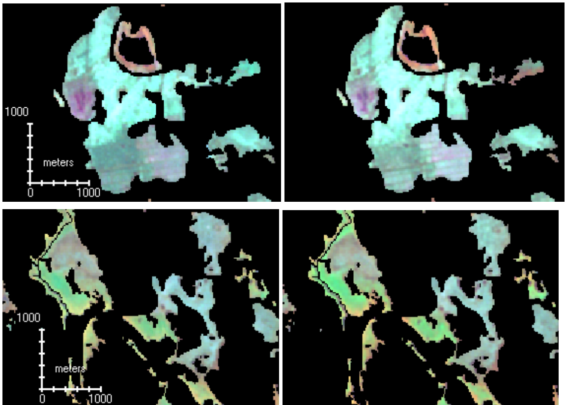
Figur 14. Jämförelse mellan de två registreringstillfällena, 1989-07-07 (bilder till vänster) och 2001-07-07 (bilder till höger) inom grönt scenpar, där både fenologi och väderförhållanden är likvärdiga vid de båda tillfällena.
