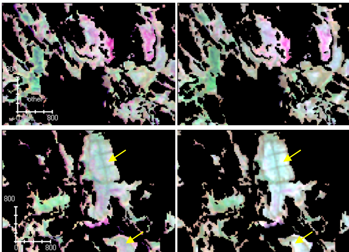
Figur 17. Jämförelse mellan de två registreringsstillfällena, 1989-08-22 (bilder till vänster) och 2001-07-05 (bilder till höger) inom rosa scenpar. Gul pil visar på myrar som är torrare 2001 än 1989.
