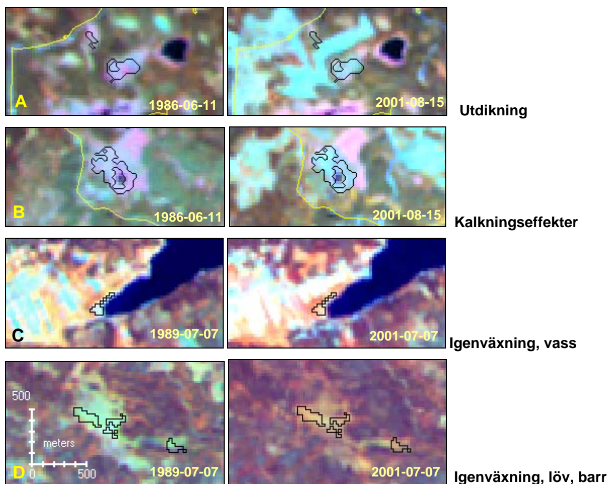
Figur 24. Exempel på förändringar som detekteras. A-B = förändringar i bottenkiktet, C-D ökad biomassa/igenväxning. Förändringarna är verifierade i fält.
