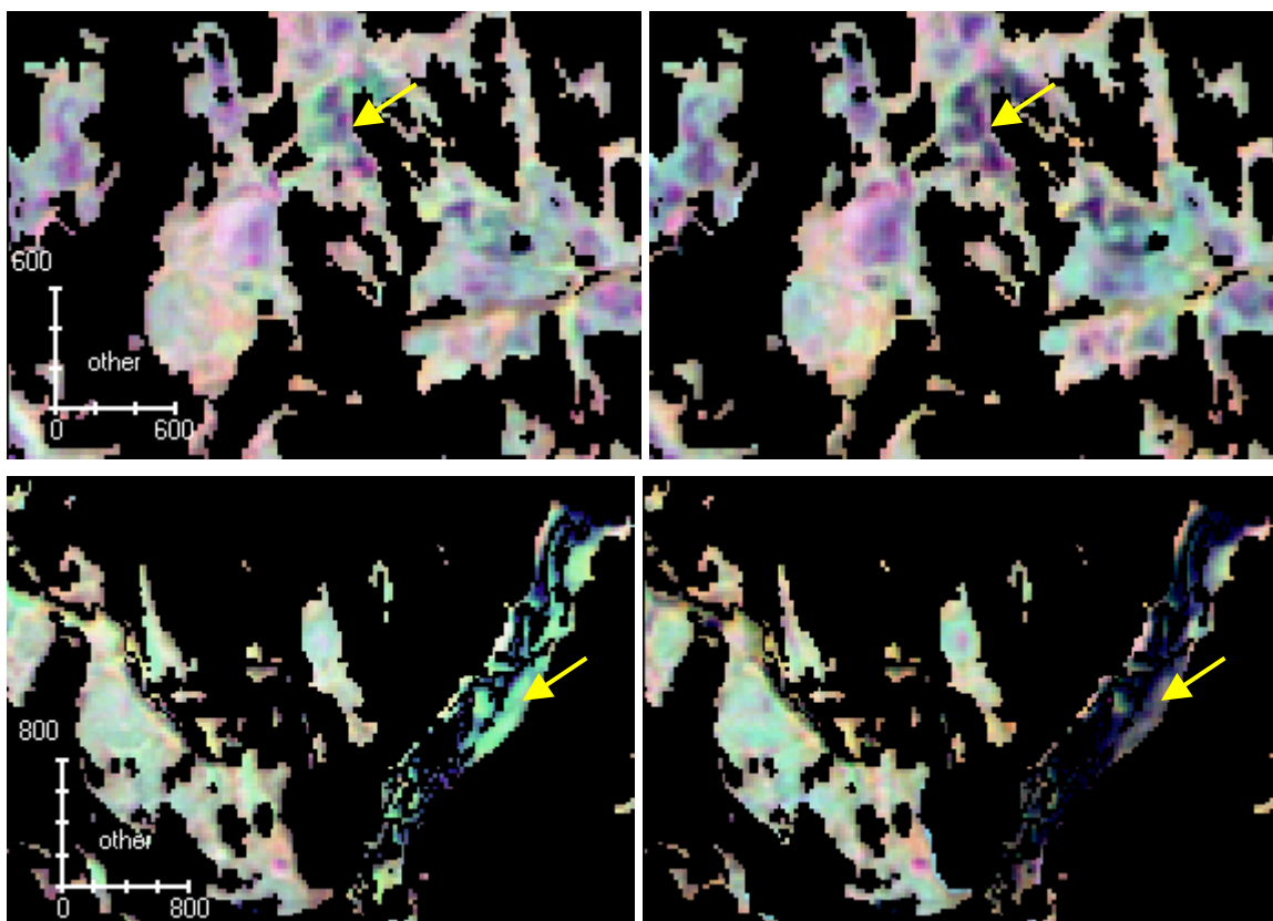
Figur 18. Jämförelse mellan de två registreringsstillfällena, 1989-08-22 (bilder till vänster) och 2000-07-28 (bilder till höger) inom rött scenpar. Gul pil visar på myrar som är blötare 2000 än 1989.
