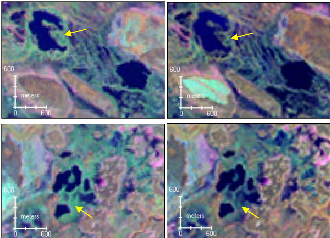
Figur 20. Exempel på skillnader mellan de två registreringstillfällena över Norrbotten, 1987-08-10 (bilder till vänster) och 2002-07-29 (bilder till höger), som främst beror på skillnader i nederbörd mellan åren.
