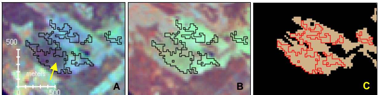
Figur 54. Exempel på förändringar som fallit ut inom delresultatet ”förändringar av bottenskikt/fältskikt” inom blått scenpar som är orsakad av den extrema torka som föregick registreringen den 5 juli 2001. Gul pil visar plats för foto i figur 55. A. 1986-06-13 B. 2001-07-05 C. Myrmask från terrängkartan, beige = öppen brunmyr.
