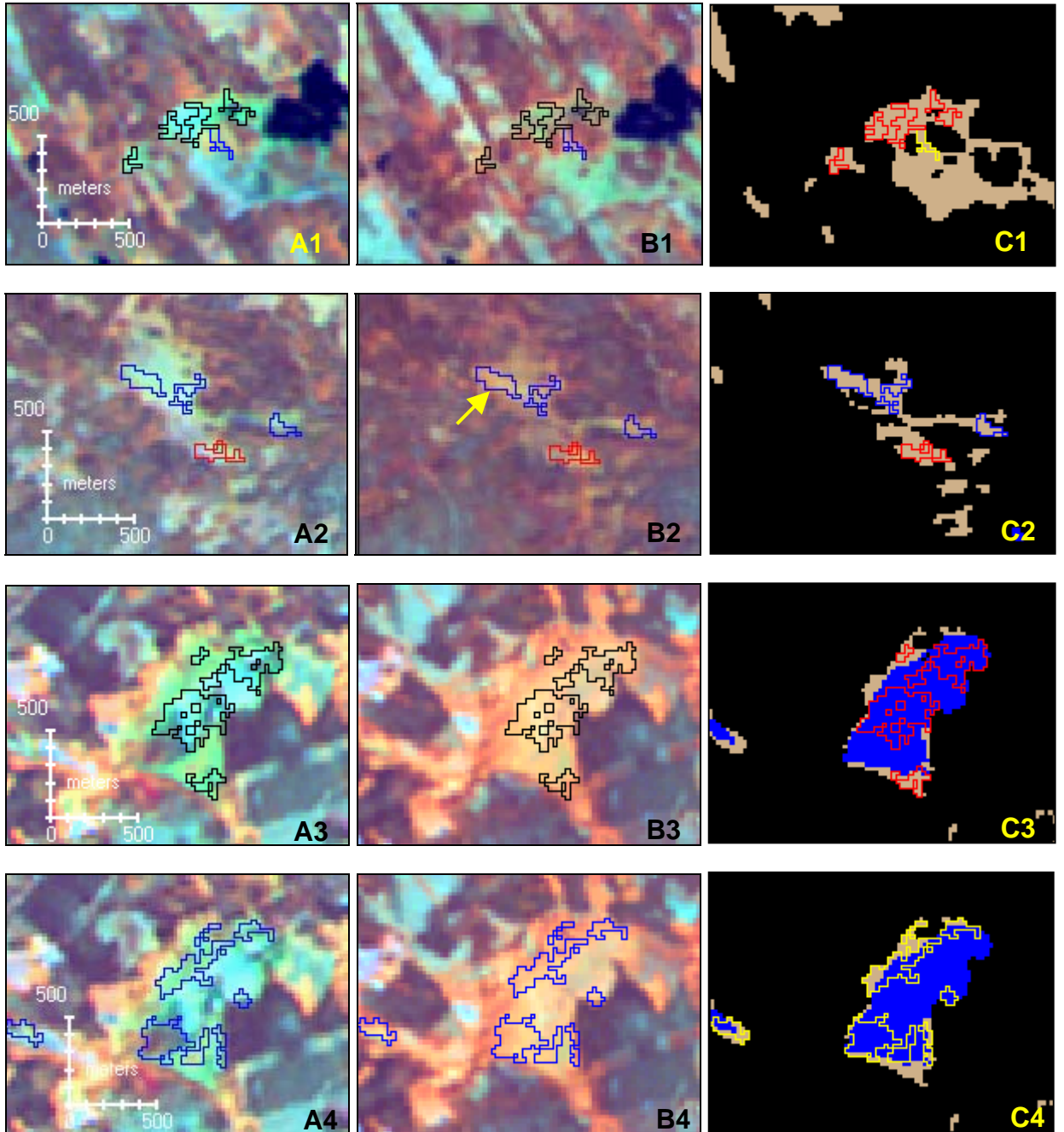
Figur 52. Exempel på förändringar som fallit ut inom delresultatet "ökad biomassa/igenväxning–3/2-kvot" samt "ökad biomassa/igenväxning–4/3-kvot" inom blått scenpar. A1-yltor. Igenväxning, svarta polygoner (3/2-kvot), blå polygon (4/3-kvot). A2-yltor. Igenväxning, blå polygon (4/3-kvot), röd polygon (fallit ut i båda förändringsmängderna). Gul pil visar plats för foto i figur 53. A3 och A4-yltor. Svårbedömt om förändringarna är av fenologisk karaktär eller en reell igenväxning. A3-yltor = 3/2-kvot, A4-yltor = 4/3-kvot. A. 1986-06-13 B. 2001-07-07 C. Myrmaskerna från terrängkartan, beige = öppen brunmyr, blått = öppen blåmyr.
