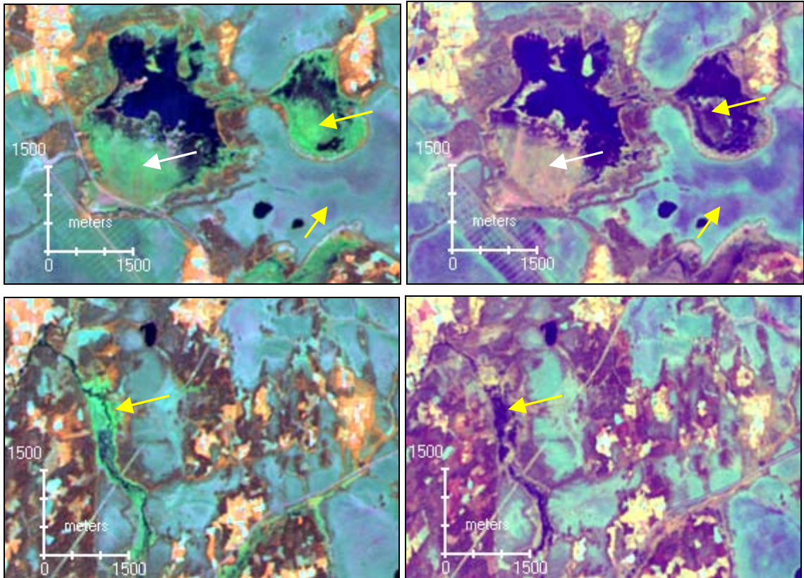
Figur 19. Exempel på skillnader mellan de två registreringstillfällena, 1985-06-01 (bilder till vänster) och 2002-07-10 (bilder till höger) över 6DSO/6ESV, som både beror på fenologiska skillnader (vegetationens utveckling, vit pil) och skillnader i nederbördsförhållanden (gula pilar).
