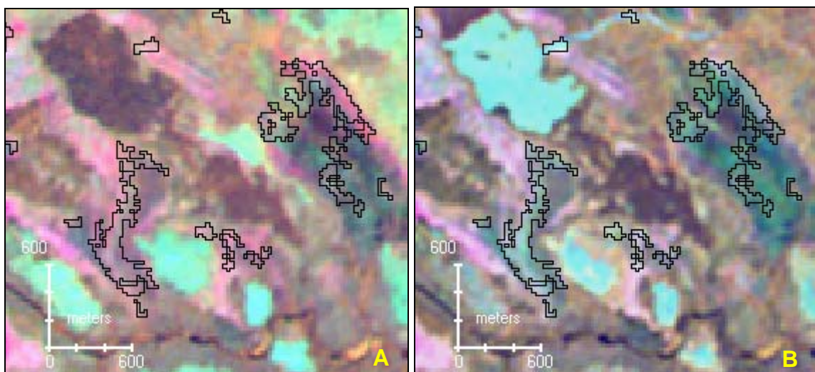
Figur 71. Exempel på några arealsmässigt stora förändringar inom delmängden "förändrat botten/fältsikt". De större ytorna utgör tillsammans ca 34 ha. A. 1987-08-10. B. 2000-07-29.
