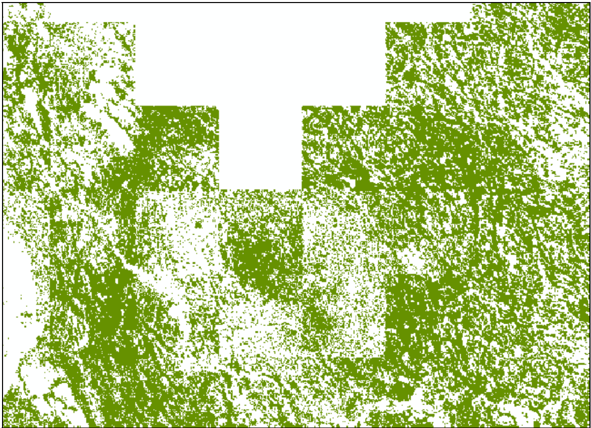
Figur 3. Fördelning av skogsklädd myr inom de olika topografiska kartbladen (terrängkartan, skala 1:50 000) över del av norra Dalarna och Gävleborgs län.
