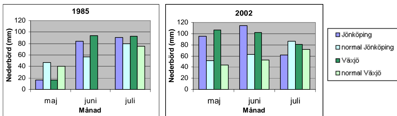
Figur 11. Månadsnederbörd för Jönköping och Växjö meteorologiska stationer för maj - juli de år som använda satellitbilder registrerats.
