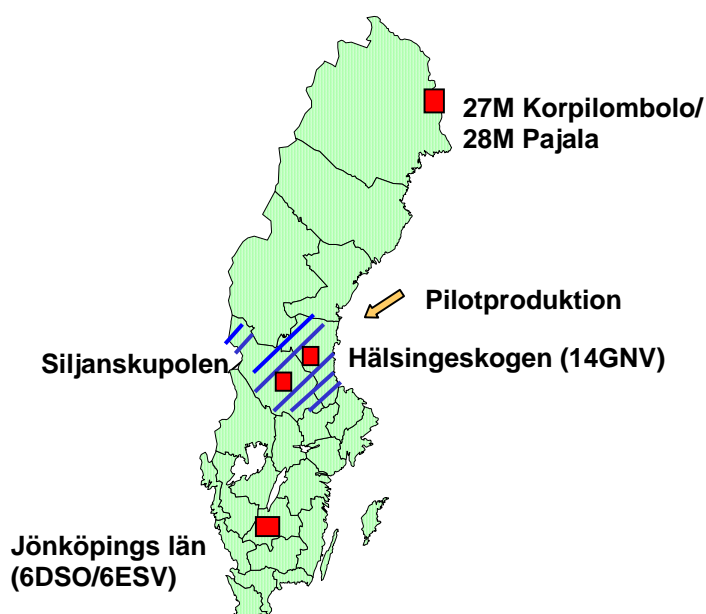
Figur 1. Studieområden och område för pilotproduktion.
