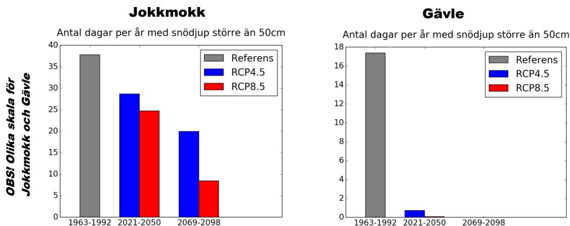
Figur 5 Medelvärde för antal dagar per år med snödjup över 50 cm för referensperioden (1963-1992), mitten av seklet (2021-2050) samt för slutet av seklet (2069-2098) i Jokkmokk respektive Gävle.
