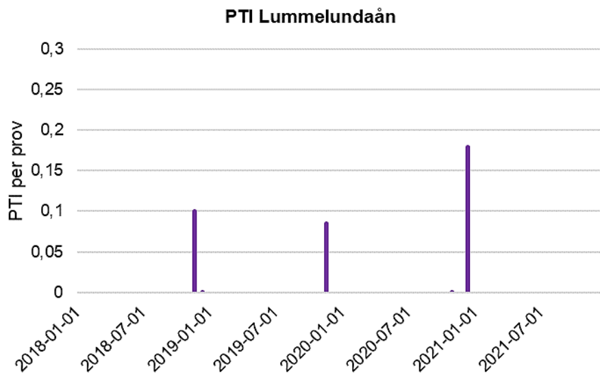
Figur 16. PTI per prov för Lummelundaån.
