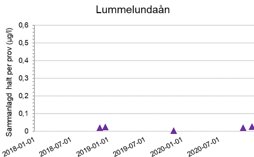
Figur 13. Sammanlagd halt per prov för Lummelundaån (µg/l).
