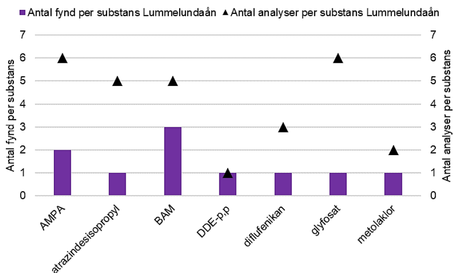
Figur 15. Antal fynd per substans och antal analyser per substans för Lummelundaån för perioden 2016-2021.
