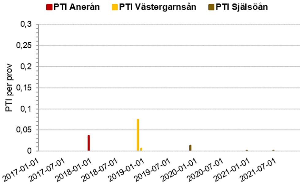
Figur 20. PTI per prov för Anerån (röd), Västergarnsån (gul), Själsoån (brun).
