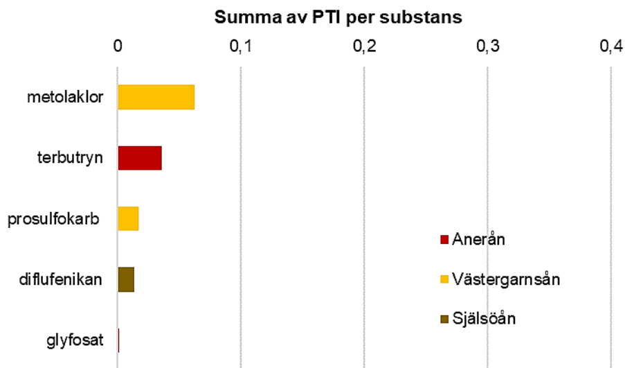
Figur 21. Enskilda substansers bidrag till PTI för Anerån (röd), Västergarnsån (gul) och Själsoån (brun) för åren 2016-2021. Substanser med bidrag till PTI ner till 0,001 redovisas i figuren.
