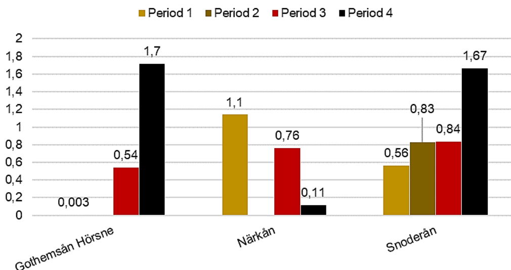
Figur 28. PTI per prov för TIMFIE prover period 1-4 för Gothemsån Hörsne, Närkån och Snoderån. Notera att endast Snoderån hade provtagare utsatt i period 2. För noggrannare information om period 1-4 se Tabell 6.
