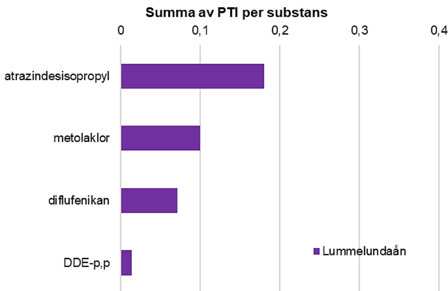
Figur 17. Enskilda substansers bidrag till PTI för Lummelundaån för åren 2016-2021. Endast substanser med bidrag mer än 0,005 syns i figuren.
