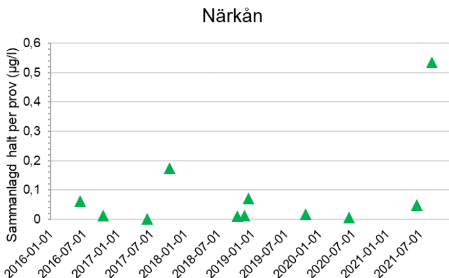
Figur 10. Sammanlagd halt per prov (µg/l) för Närkån.
