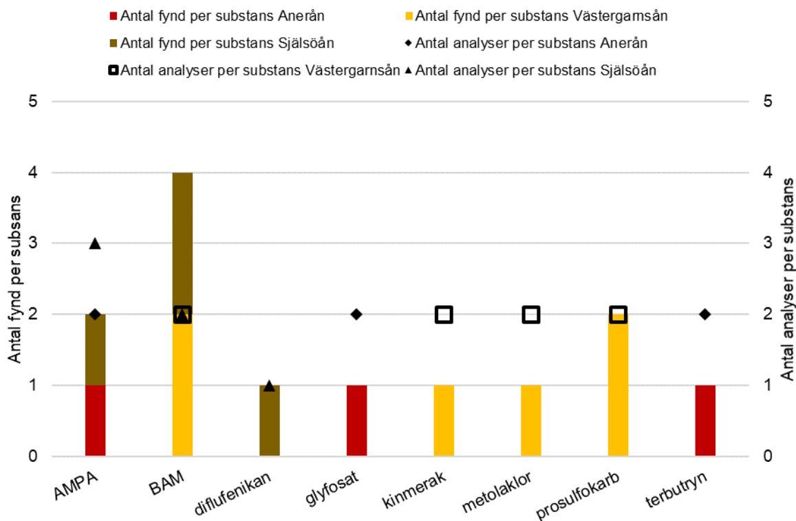
Figur 19. Totalt antal fynd per substans (hela stapeln) samt antal fynd och antal analyser per provplats för Anerån (röd; romb), Västergarnsån (gul; fyrkant) och Själsoån (brun; triangel) per substans för åren 2016-2021.
