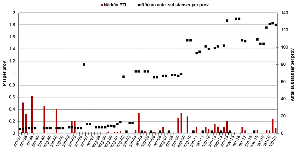
Figur 23. PTI per prov och antal analyserade substanser per prov för Närkån 1987-2021.
