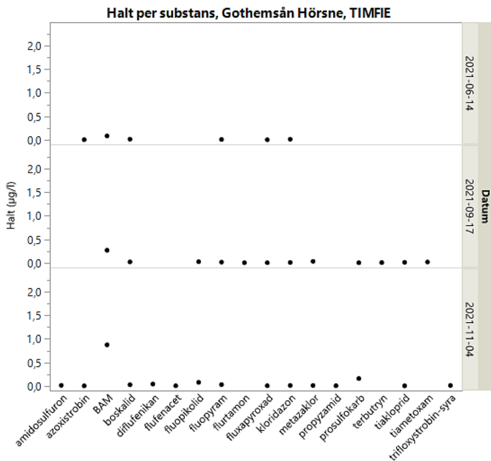
Figur 25. Halt per substans för TIMFIE-provtagning i Gothemsån Hørsne. Period 1 (7/6-14/6), period 3 (10/9-17/9), period 4 (28/10-4/11). Datumet i figuren anger sista datumet för perioden.
