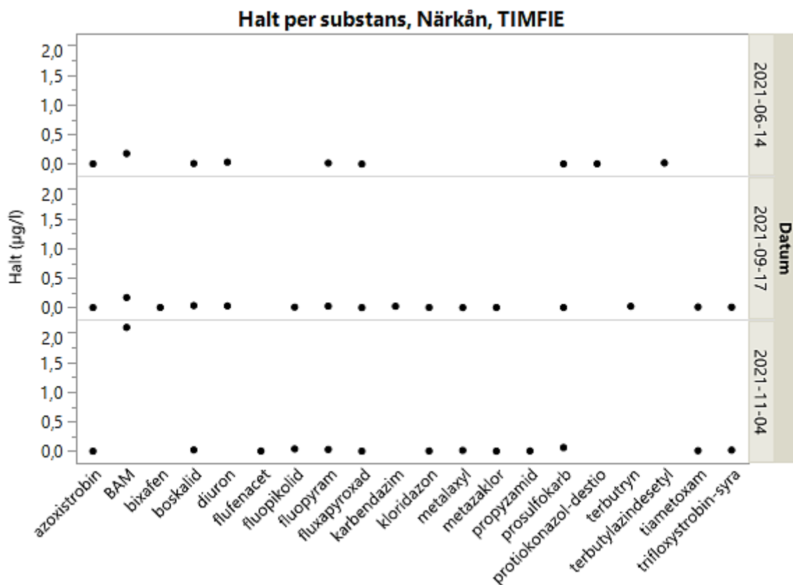
Figur 26. Halt per substans för TIMFIE-provtagning i Närkån. Period 1 (7/6-14/6), period 3 (10/9-17/9), period 4 (28/10-4/11). Datumet i figuren anger sista datumet för perioden.
