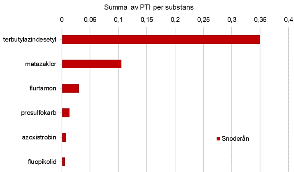
Figur 9. Enskilda substansers bidrag till summan av PTI för åren 2016-2021 för Snoderån. Figuren visar endast substanser som bidrar med minst 0,005 till PTI, varför Snoderån Borum ej syns i figuren.
