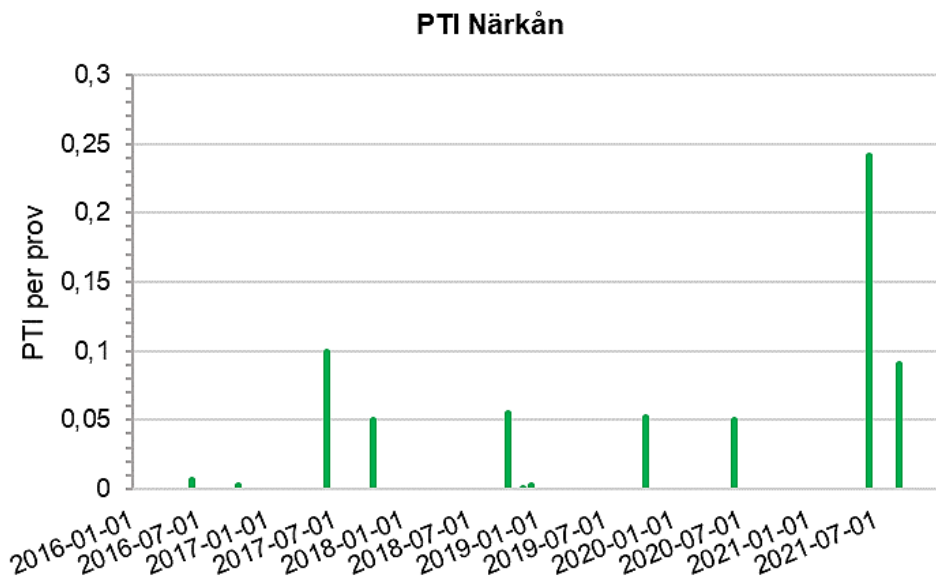
Figur 12. PTI per prov för Närkån.
