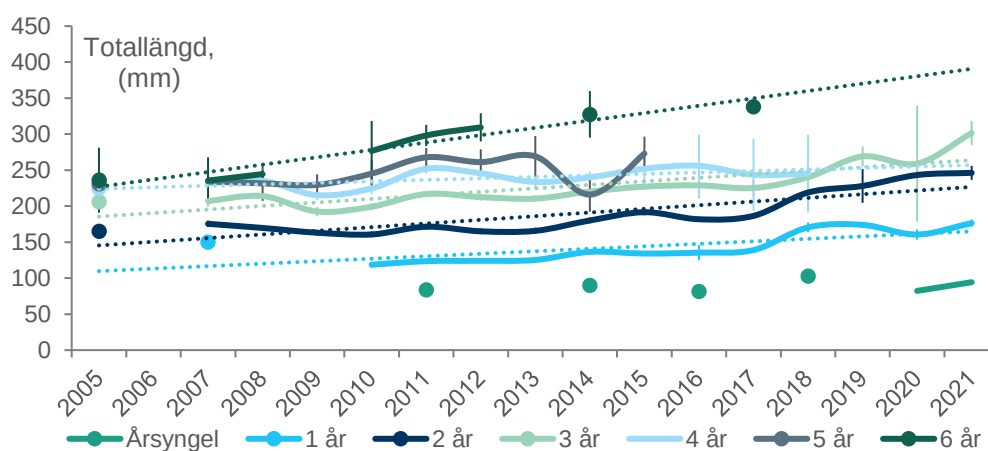
Figur 7. Medellängd för 0–6 år gamla abborrhonor i Asköfjärden. Data saknas från 2006. 2005–2009 provtogs endast abborrar i längdgrupper 15–25 cm. Vertikala linjer anger 95 % konfidensintervall. Streckade linjer anger signifikanta trender ( p < 0,05 ) för tidsperioden 2010–2021.
