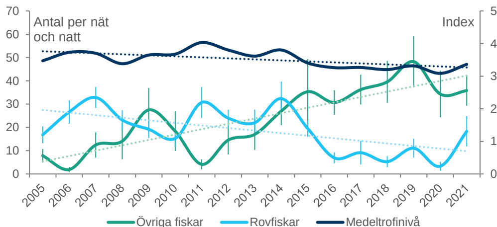
Figur 6. Fångst per nät och natt av rovfiskar och icke-rovfiskar, samt Trofisk medelnivå. Vertikala linjer anger 95 % konfidensintervall. Den trofiska medelnivån är ett index och visas på den högra y-axeln. Indexet har inga spridningsmått eftersom det beräknas över hela fångsten. Streckad linje anger signifikant trend ( p < 0,05 ).
