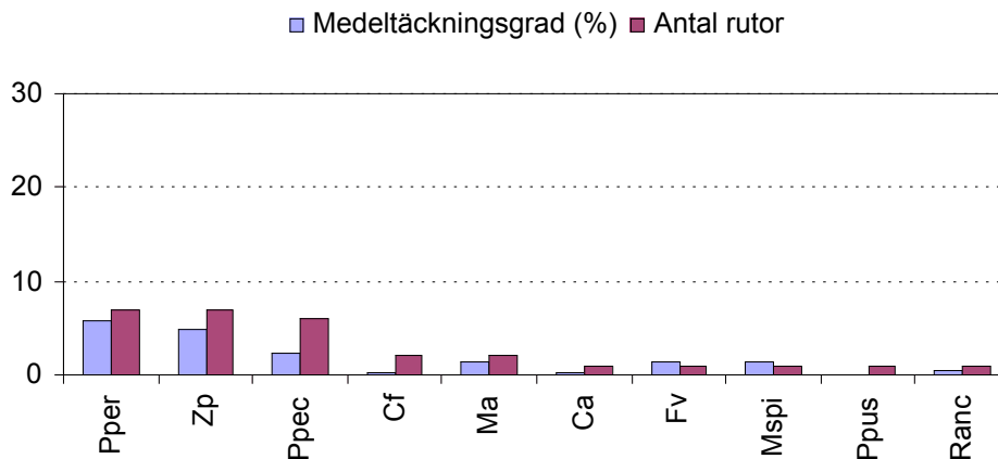
Figur 27. Resultat från vegetationskarteringen i viken mellan Lilla Risten och Måsören. Totalt inventerades 27 rutor. Förkortningarna ges i tabellen som inleder resultatkapitlet.
