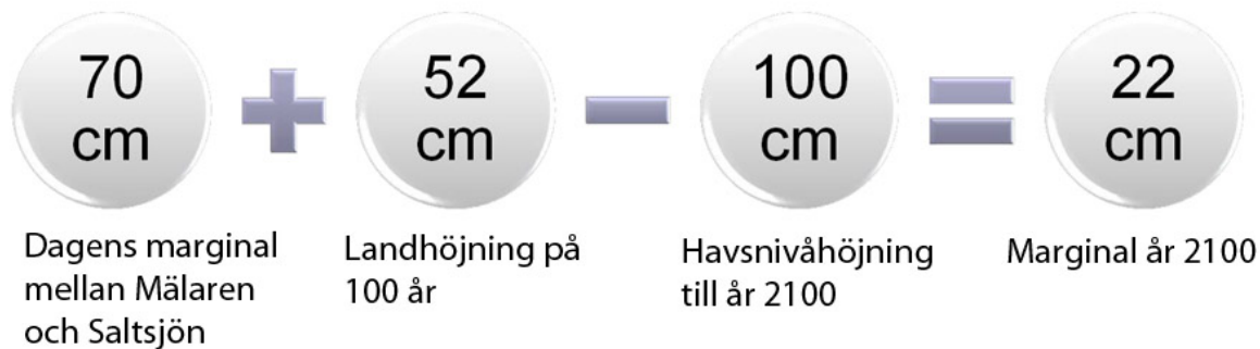
Figur 6. Mälarens marginal till Saltsjön om havet stiger med 1 meter vid normalt vattenstånd.
