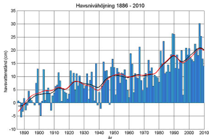
Figur 4. Havsvattenståndets (årsmedelvärden) förändring korregerade för den absoluta landhöjningen runt Sveriges kuster (baserat på 14 mätstationer) jämfört med 1886 års nivå. Stockholm följer medelvärdet för Östersjön. Den röda och svarta linjen visar gauss-filtrerade¹ årsvärden för Stockholms respektive alla stationer (Hammarklint, 2011).
