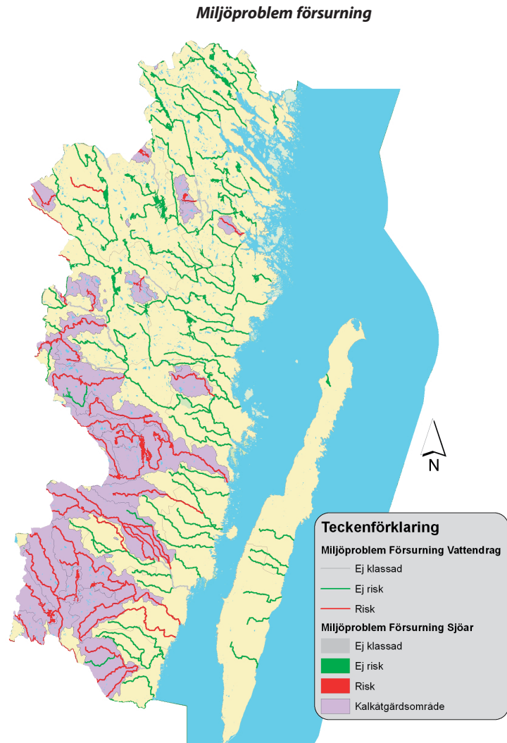
Figur 6. Miljöproblem förurning klassad utifrån EU:s vattendirektiv
