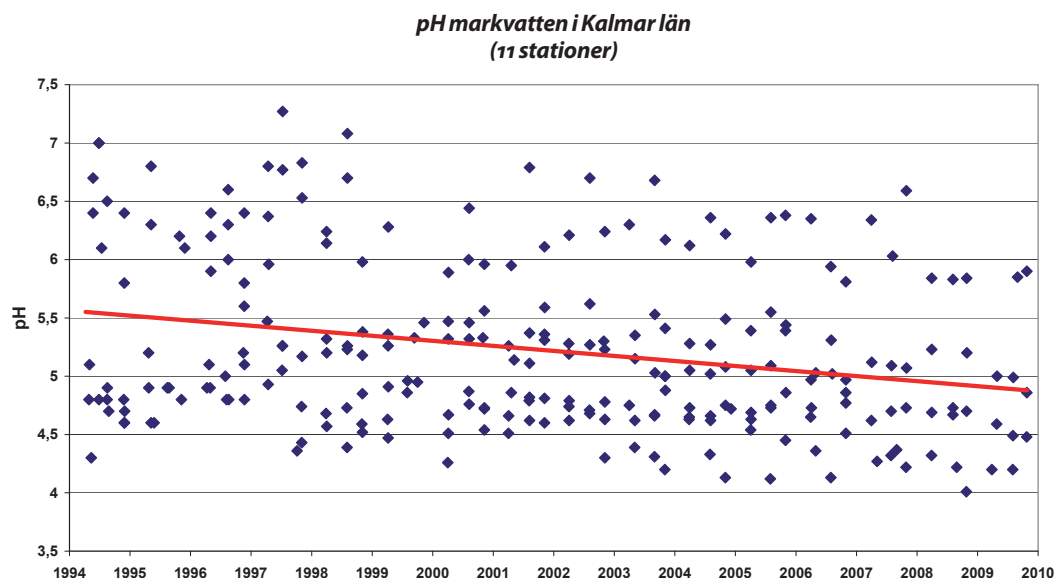
Figur 4. SvavelpH-mätningar i markvatten vid elva stationer inom Kalmar län. Mätningarna genomförda inom Krondroppsnätet.
