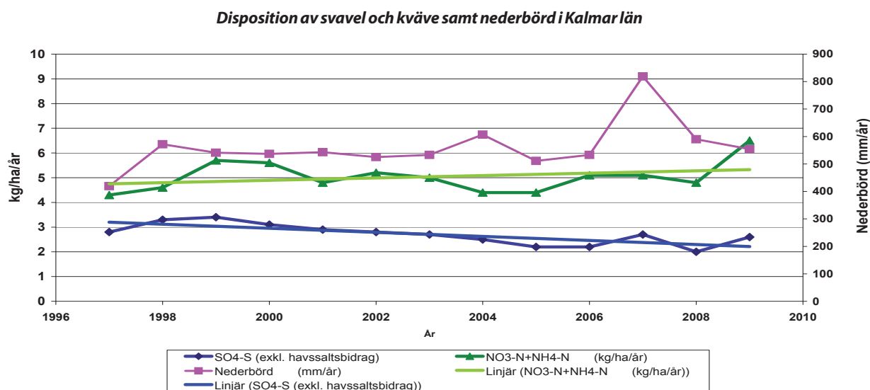
Figur 1. Resultat från Krondroppsnätets öppet-fältsmätningar i Rockneby, nordväst om Kalmar
