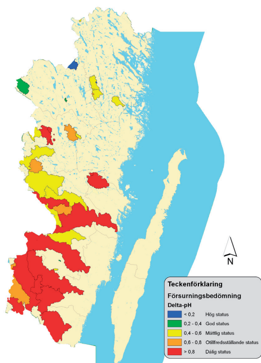
Figur 5. Påverkan av försuring vid okalkade förhållanden i kalkåtgärdsområdet
