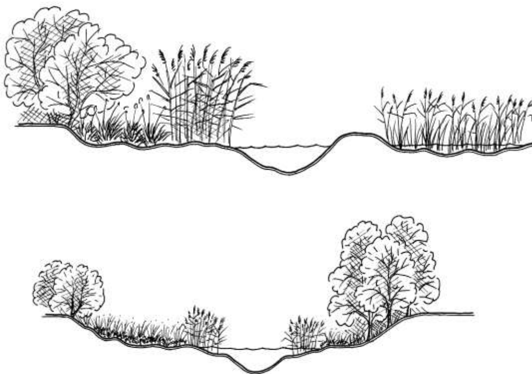
Figur 49. En högre ambitionsnivå är att etablera ett åplan genom att ”hyvla” ned kanterna i större utsträckning, etablera små våtmarker som fungerar som svämområden vid högvatten och låta kantzoner växa upp med träd och buskar . Ill. T. Nydén.
