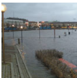
Figur 14. Lågtryck från väster trycker upp havsvatten mot kusten.
