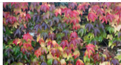
Figur 95. Vegetation absorberar vatten – Malmö.
