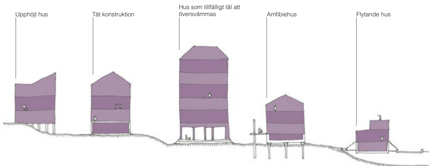
Figur 48. Översvämningssanpassade byggnader.
