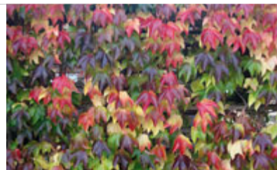
Figur 34. Vegetation absorberar vatten – Malmö.
