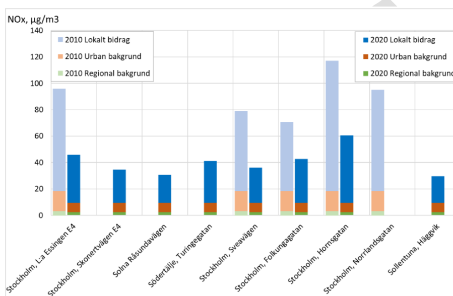
Figur 9. Årsmedelvärden av lokalt, urbant och regionalt bidrag till NO x , uppmätta vid mätstationer i länet år 2010 och 2020.
