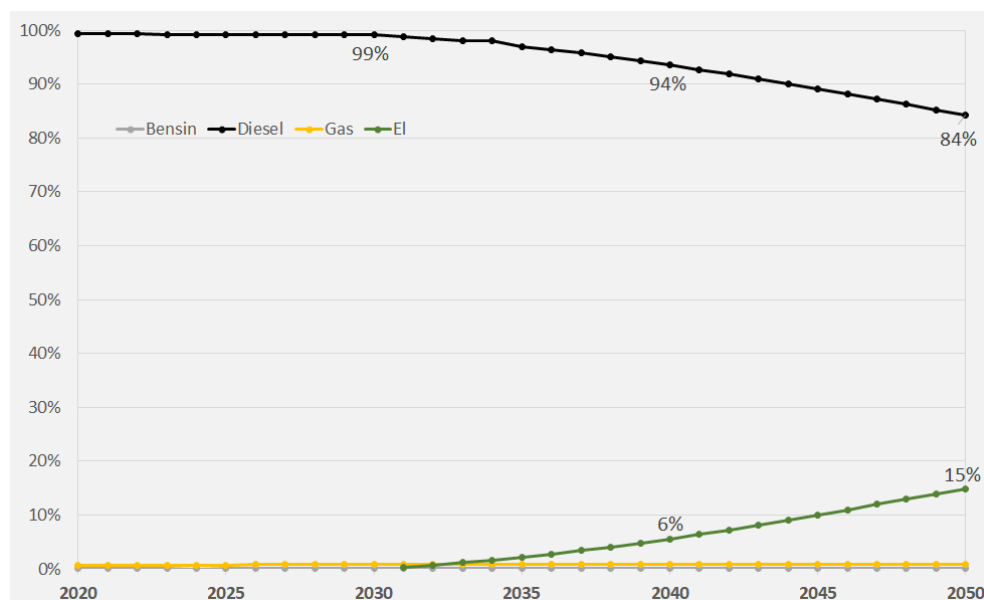
Figur 31. Nationella prognoser för fordonsammansställning för tunga lastbilar (Share of Vehicle km, Urban traffic HBEFA 4.1 år 2019).
