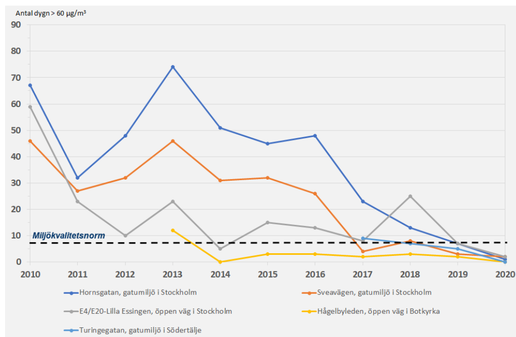
Figur 36. Trender för antal höga dygnsmedelvärden av kvävedioxid, NO 2 , (högre än normvärdet 60 µg/m³) vid olika mätstationer i Stockholms län, från år 2010 till år 2020 [7,8].
