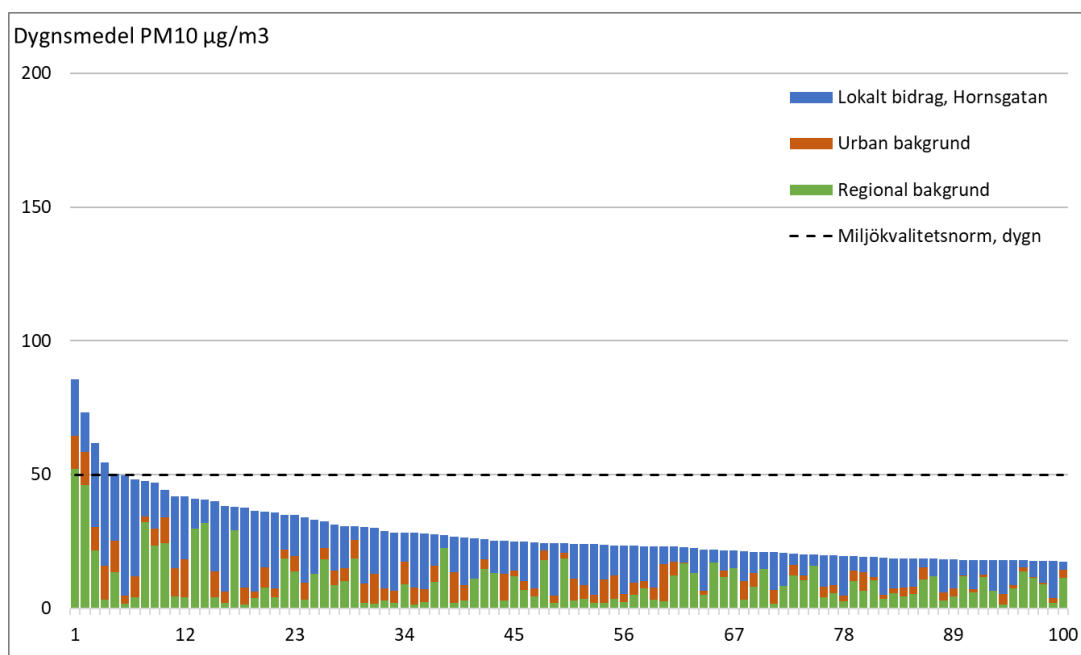
Figur 49. Fördelning av lokalt, urbant och regionalt bidrag till dygnsmedelhalten av de 100 värsta dygna av PM10 år 2020 vid Hornsgatan i Stockholm.
