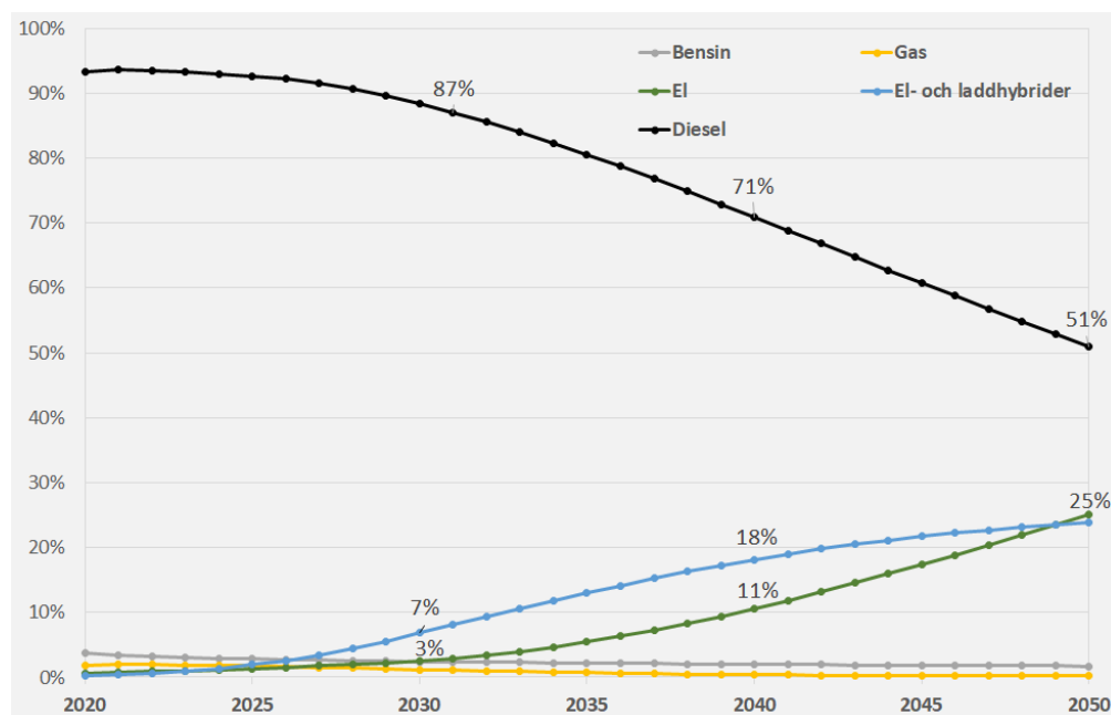
Figur 30. Nationella prognoser för fordonsammansställning för lätta lastbilar (Share of Vehicle km, Urban traffic HBEFA 4.1 år 2019).
