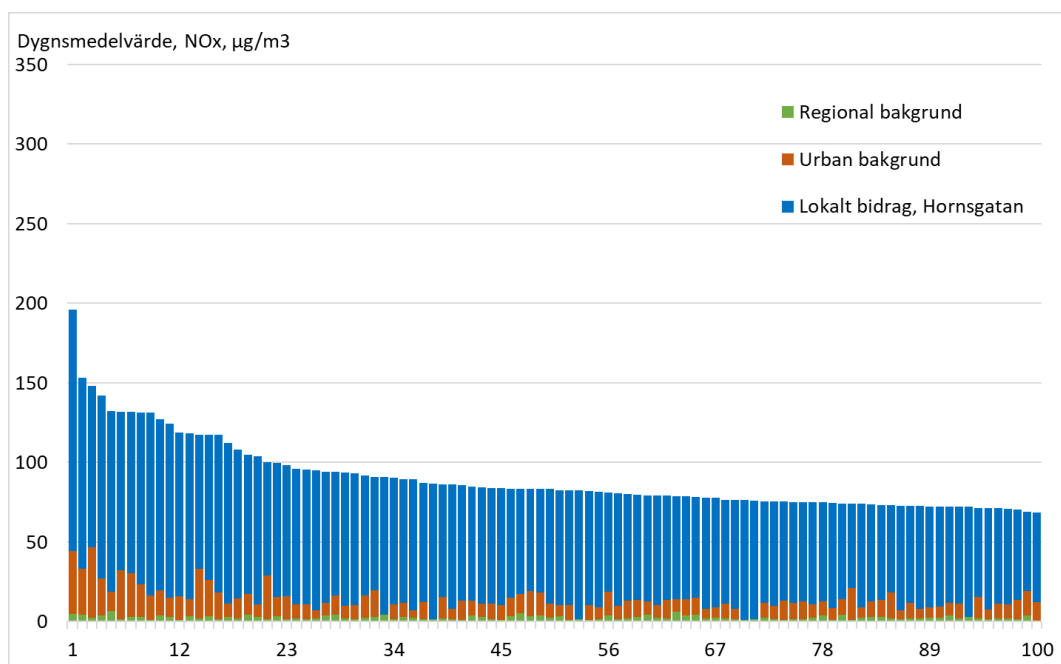
Figur 46. Fördelning av lokalt, urbant och regionalt bidrag till dygnsmedelhalten av de 100 värsta dygnen av kväveoxider, \text{NO}_x , år 2020 vid Hornsgatan i Stockholm.
