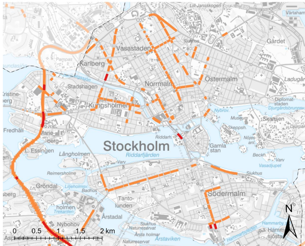
Partiklar, PM 10 dygnsmedelvärde år 2020
