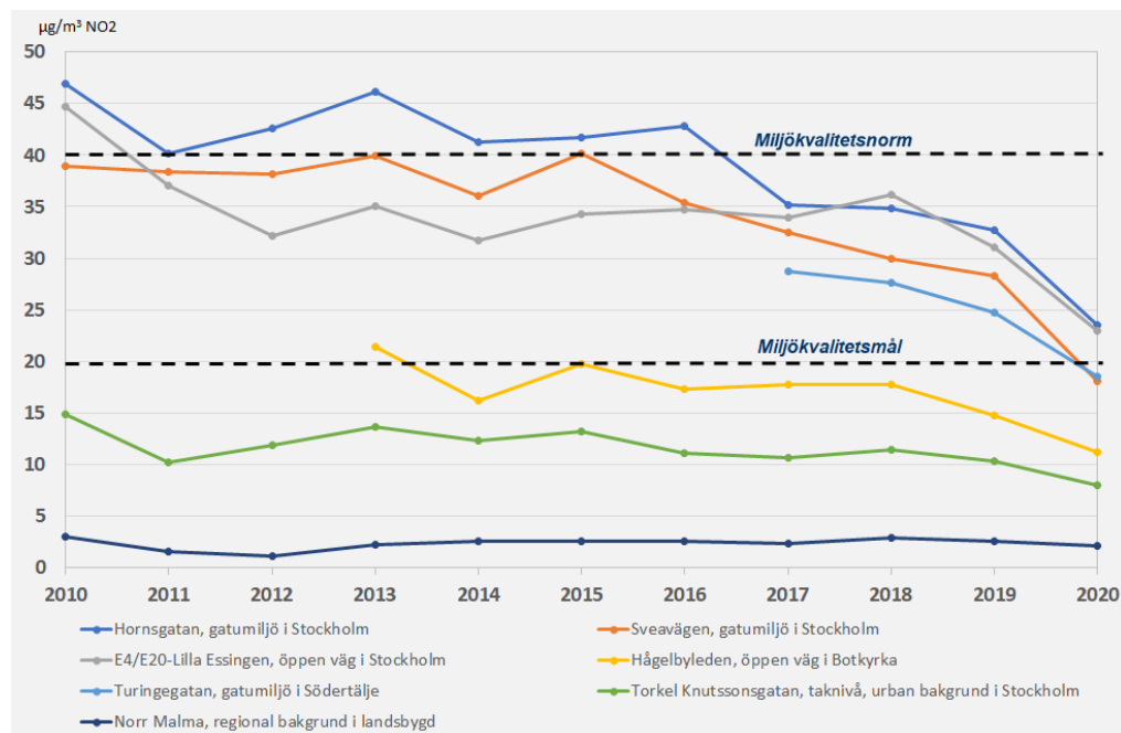
Figur 35. Trender för årsmedelvärden av kvävedioxid (NO 2 ) vid olika mätstationer i Stockholms län, från år 2010 till år 2020 [7,8].
