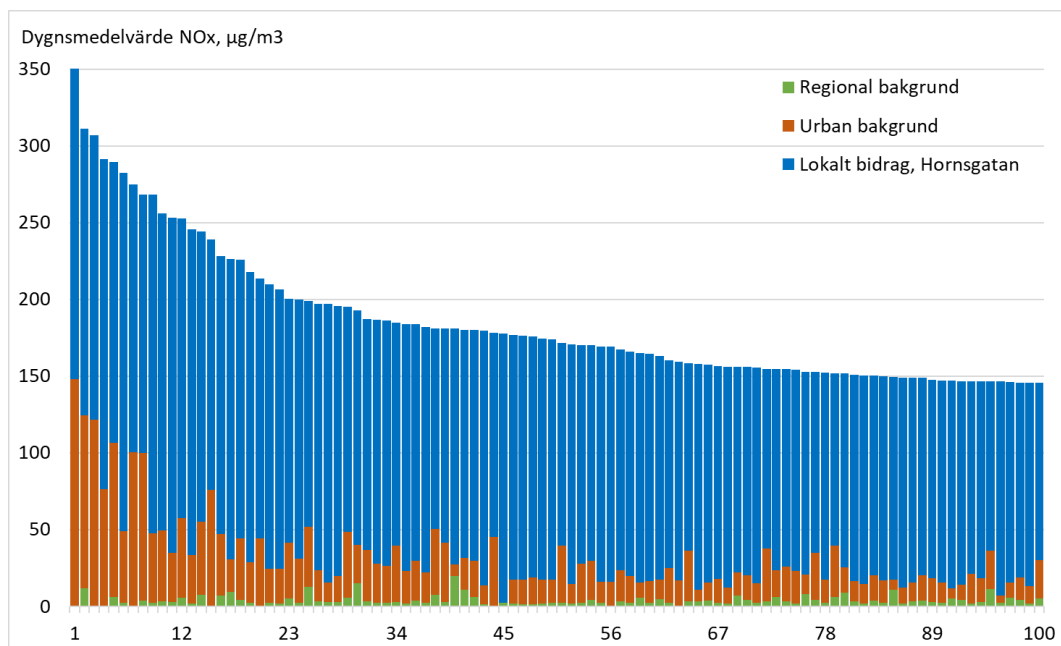
Figur 45. Fördelning av lokalt, urbant och regionalt bidrag till dygnsmedelhalten av de 100 värsta dygnen av kväveoxider, \text{NO}_x , år 2010 vid Hornsgatan i Stockholm.
