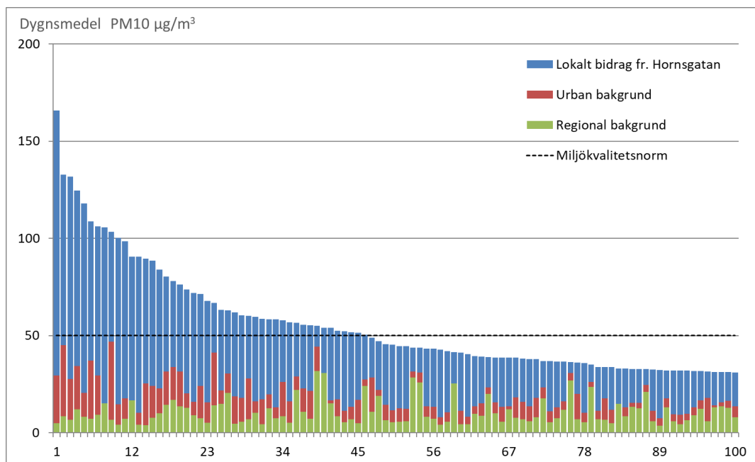
Figur 48. Fördelning av lokalt, urbant och regionalt bidrag till dygnsmedelhalten av de 100 värsta dygna av PM10 år 2010 vid Hornsgatan i Stockholm.
