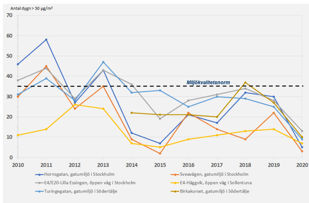
Figur 38. Trender för antal höga dygnsmedelvärden (högre än normvärdet 50 µg/m 3 ) av partiklar PM 10 , vid olika mätstationer i Stockholms län, från år 2010 till år 2020 [7,8].
