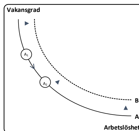
Diagram 16. Illustration över (det teoretiska) sambandet mellan vakanser och arbetslöshet, Beveridgekurvan.
