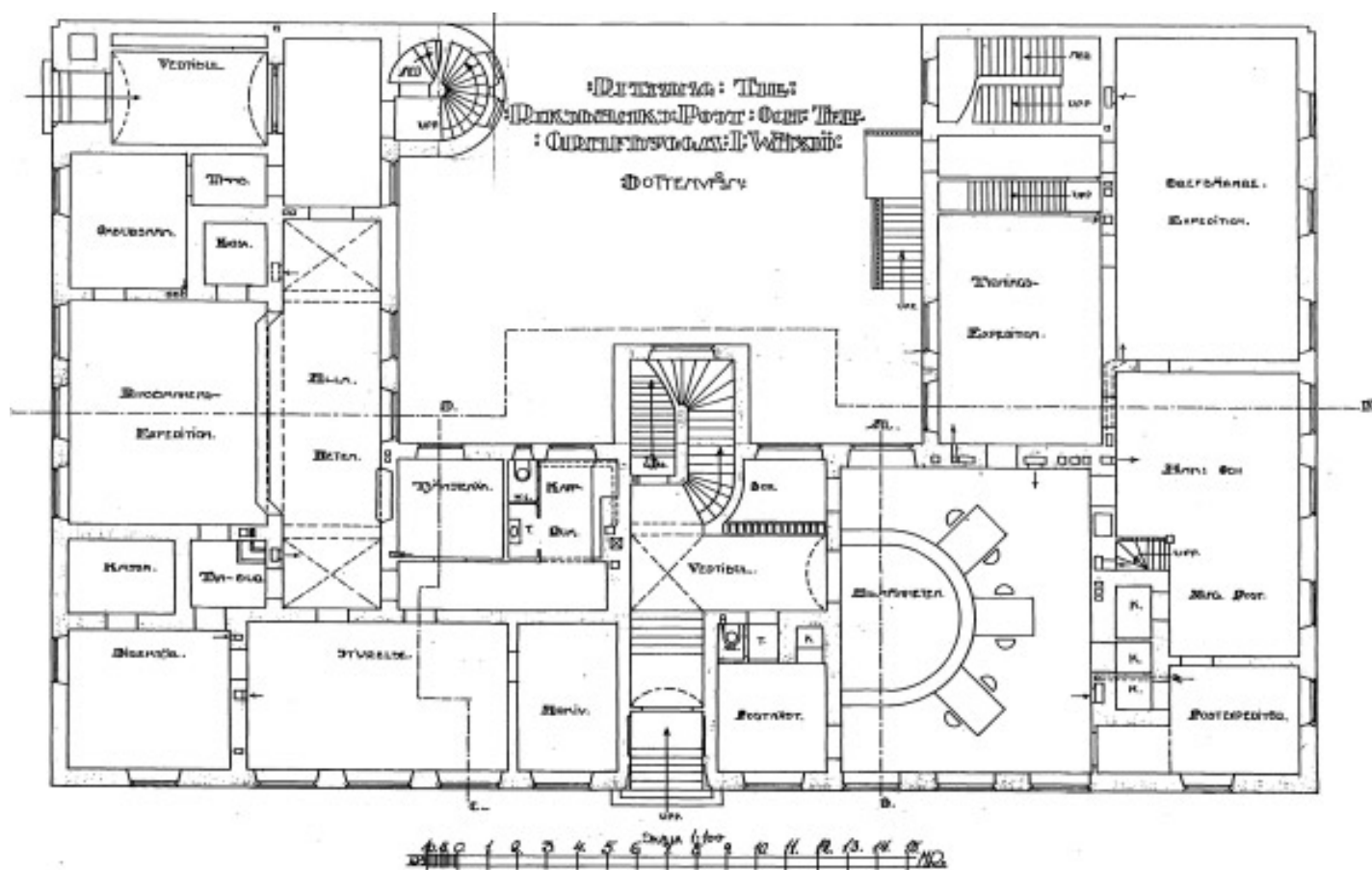
På originalritningen till bottenvåningen kan man se att lokalerna för riksbank och post var tydligt åtskilda. Foto: Stadsbyggnadskontoret, Växjö kommun.
