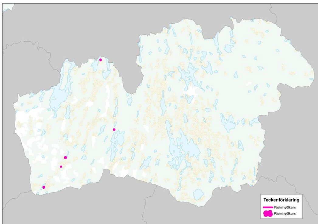
Fig 24. Kartan visar skanslämningar i Kronobergs län enligt fornlämningsregistret. Traryds (Traryd 18:1) och Kylhults skansar (Traryd 37:1) är båda daterade till 1650-tal. Hylte skans (25:1) är ej daterad, men har 15- och 1600-talets typiska stjärnform och sicksackformade vall (25:2). I Hylte socken finns ytterligare en förmodad skanslämning (26:1) av mer otydlig karaktär. I Agunnaryd socken, strax norr om sjön Möckeln, finns en förmodad skanslämning med otydlig karaktär (Agunnaryd 41.1). Tofta skans (Dörarp 38:1) är den nordligaste av Västra Kronobergs skansar, och bör därför ha haft en något avvikande funktion jämfört med de samtida skansarna i södra Lagadalen. Källa FMIS
