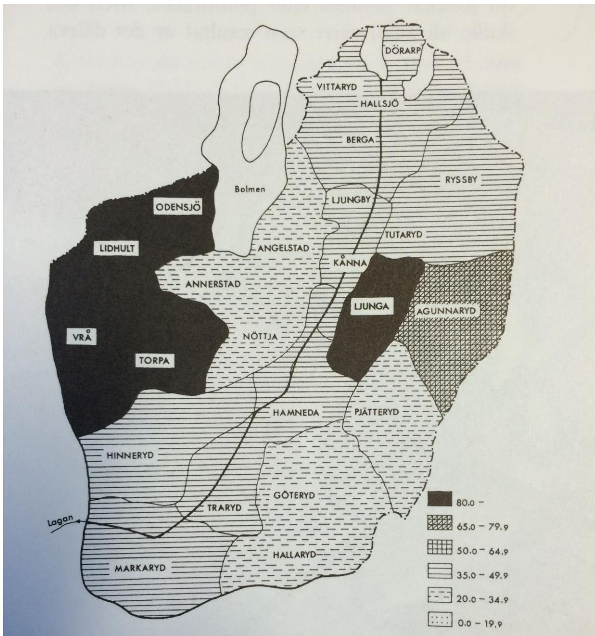
Fig 9. Kartan visar Nordiska sjuårskrigets verkningar för Sunnerbo i form av andelen gårdar som 1570 var skattebefriade till följd av härjningar och utarmning. Socknen Södra Ljunga drabbades av en systematisk ödeläggels, och socknens samtliga gårdar brändes vintern 1568. Socknarna längs med Lagastigen fick upp till 50 % skatteavkortning som en följd av deras utarmning under kriget.
