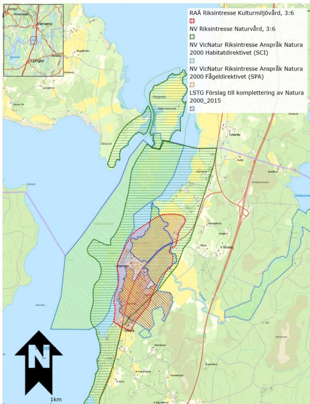
Fig 2. Överlappande riksintressen och Natura 2000-områden. Källa: LST Kronoberg, WebbGIS
